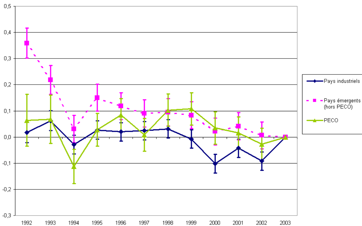
Graphique 3 : décomposition de l'effet fixe temporel par nature du marché de destination (spécification de référence)
