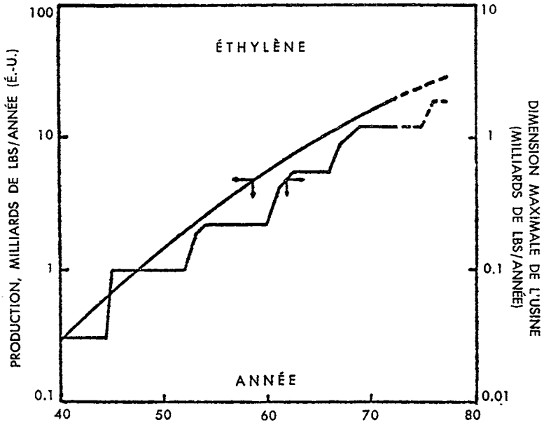
CROISSANCE EN ESCALIER DE LA DIMENSION DE LA PLUS GRANDE USINE D'ÉTHYLÈNE (É.-U.)
