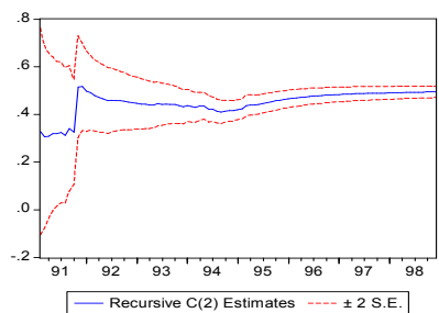
Fig. 1. Estimativa por Mínimos Quadrados Recursivo (MQR) de \varphi_1 da PCJ, jun./1990 a dez./1998
