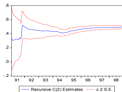
Fig. 1. Estimativa por Mínimos Quadrados Recursivo (MQR) de \varphi_1 da PCJ, jun./1990 a dez./1998
