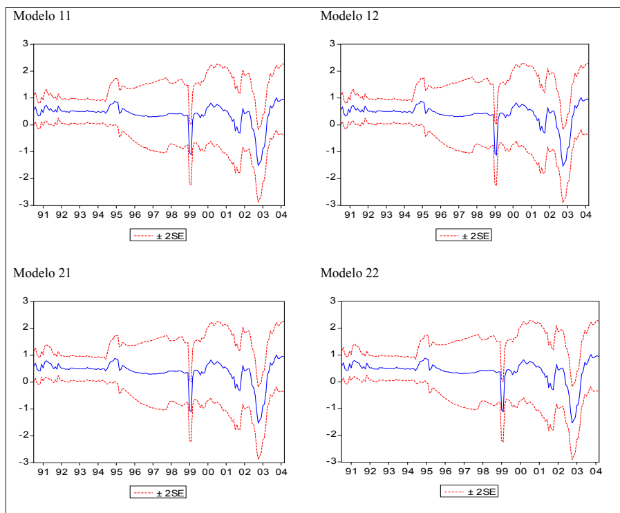
Fig. 2. Estimativas suavizadas por Filtro de Kalman de \varphi_1 da PCJ de jun./1990 a mar./2004
