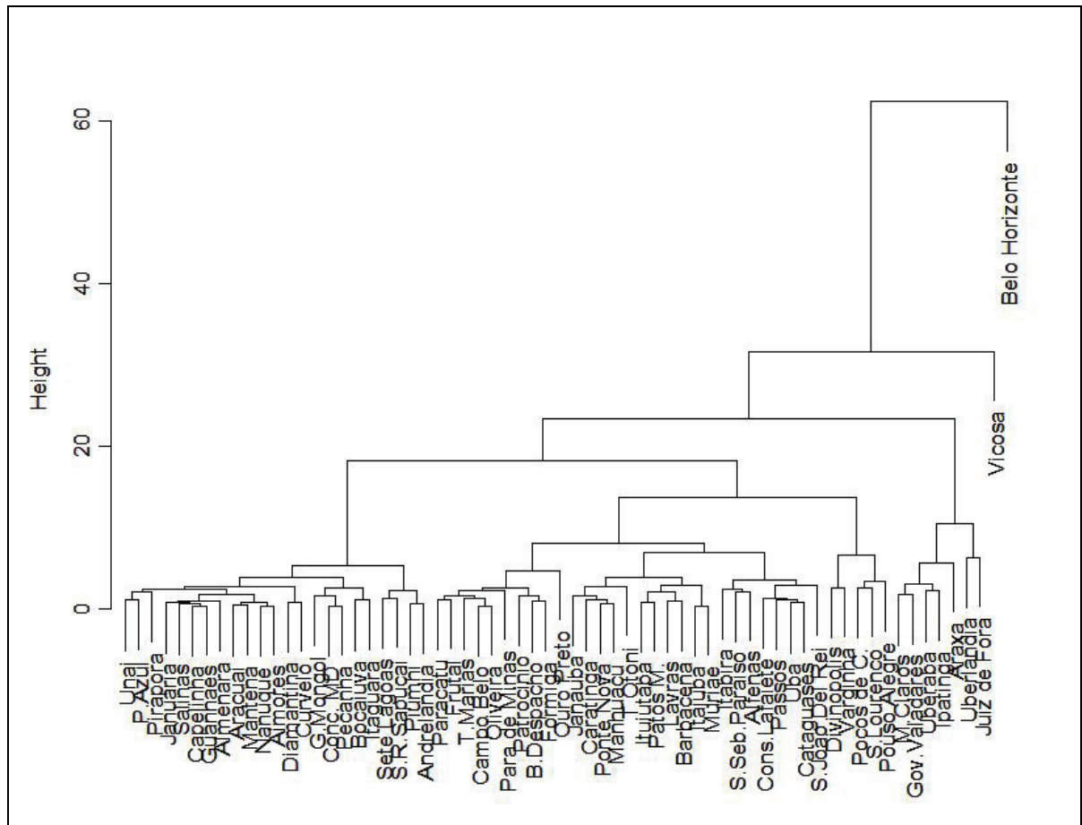
Figura 04 – Clusters – Agglomerative Hierarchical (distância euclidiana) - 2007
