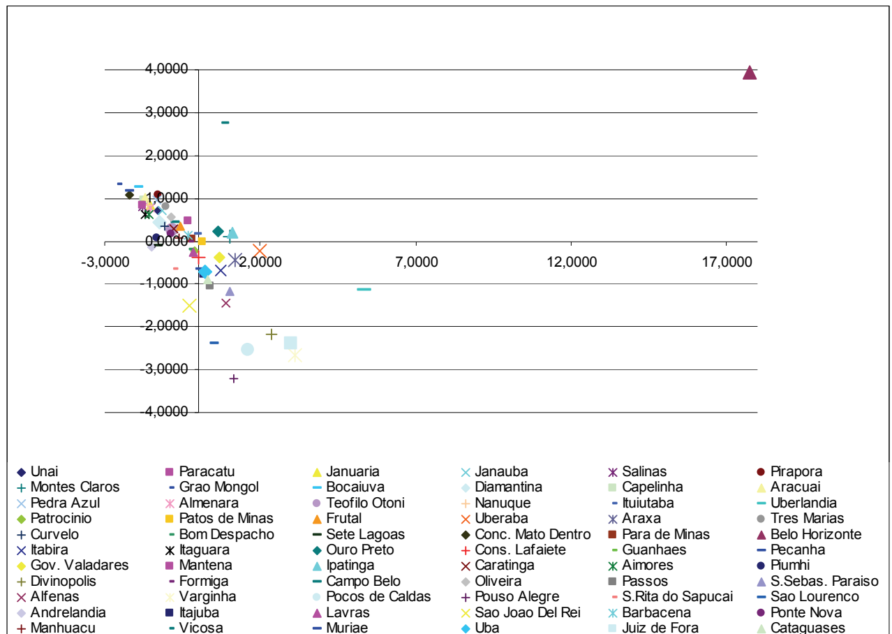
Figura 03 – Distribuição das microrregiões de acordo com os dois primeiros componentes principais
