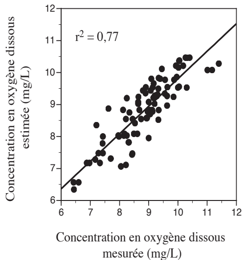
Figure 6 Relation entre la concentration en oxygène dissous estimée et mesurée (mg/L) pour les sept cycles diurnes aux stations Hurons et RSC2.
