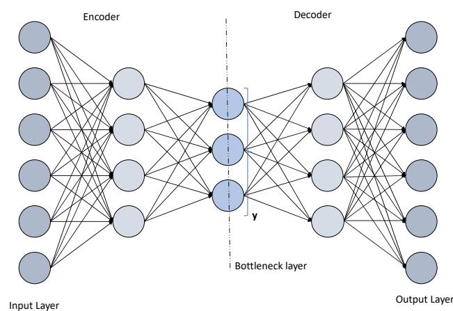
Figure 15. Deep autoencoder (DAE) [105].
