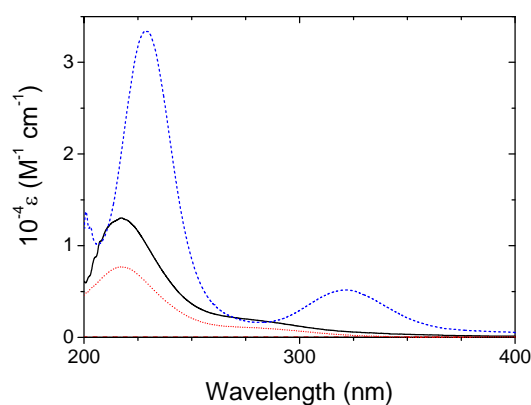
Fig. 3 Spectra of AuCl 4 - at pH 5.0, [NaCl]= 0.0 M, T= 25°C: (•••) water, (—) SDS 0.04 M, (--) DTAC 0.04M.
