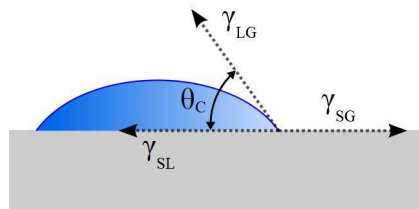
Figure 2.3: Ligne de contact et angle de contact
