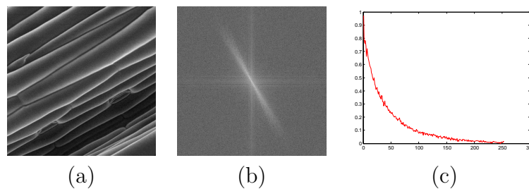
Figure 2.16: Exemple de calcul du DGF (a) Image originale, (b) Transformée de Fourier, (c) Allure du vecteur caractéristique ou DGF
