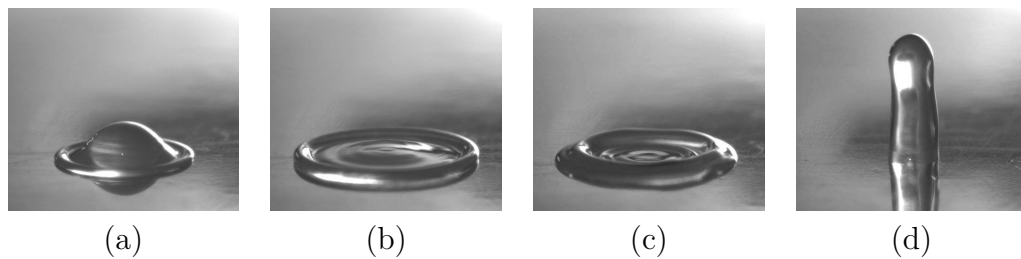
Figure 2.1: Les différentes phases lors de l'impact (a) la phase cinématique, (b) la phase d'étalement, (c) la phase de recul, (d) la phase finale [ Roisman et al., 2002 ]
