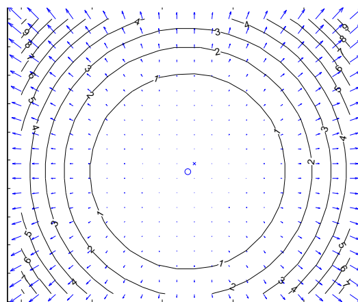
Figure 3.6: Modèle complet de distorsion de l'objectif de 50 mm
