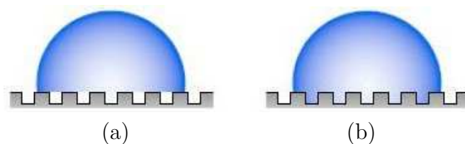
Figure 2.5: Selon [ Quéré and Reyssat, 2008 ], les modèles de Cassie-Baxter (a) et de Wenzel (b)
