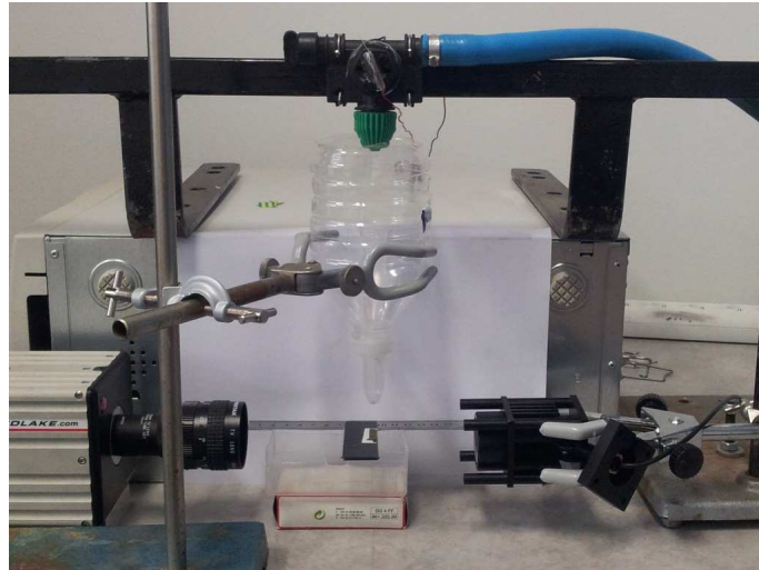
Figure 3.17: Système complet
