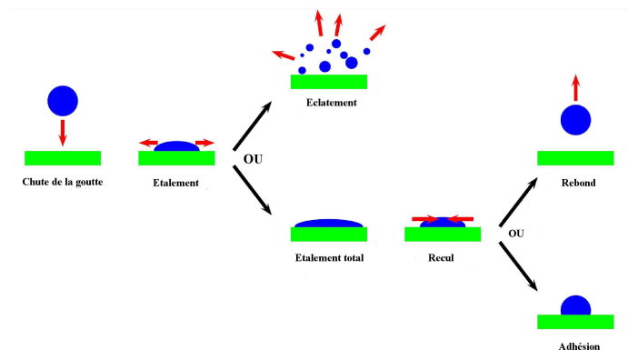
Figure 2.2: Les comportements possibles d'une goutte lors de l'impact
