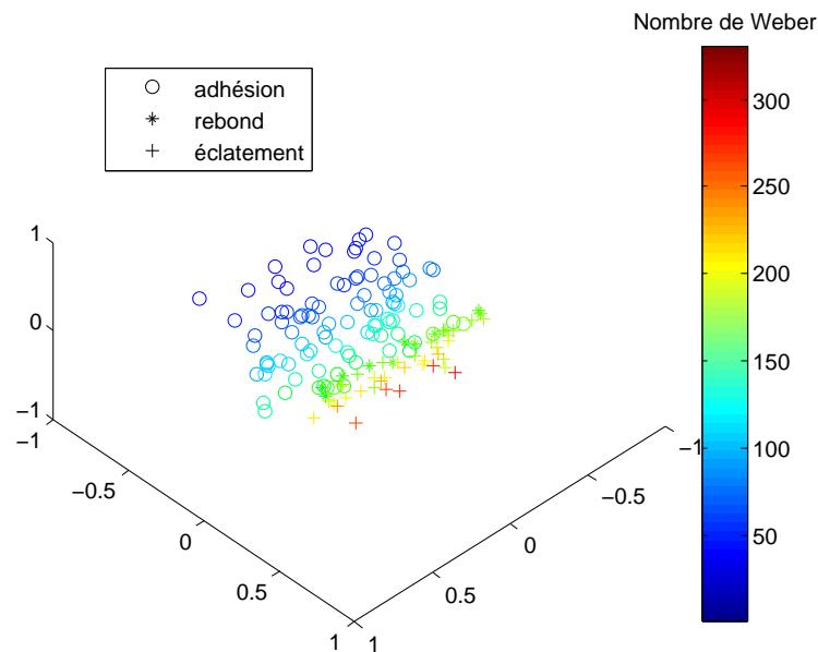
Figure 4.17: Illustration de l'influence du nombre de Weber sur le comportement
