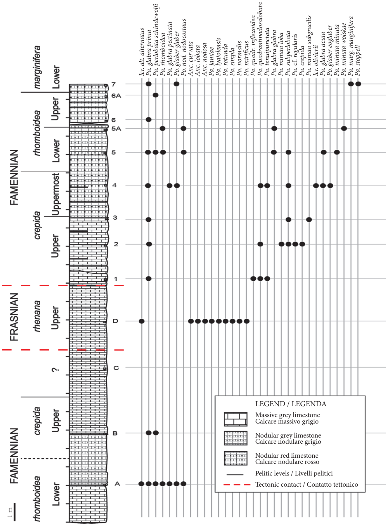
Fig. 3 - Stratigraphic log of the Pizzul West section and conodont distribution - Colonna stratigrafica e distribuzione dei conodonti nella sezione Pizzul Ovest.
