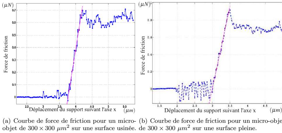
FIGURE 4.23 – Exemple de courbe de friction obtenue sur les deux types de surfaces pour un micro-objet de 300 \times 300 \mu\text{m}^2 .
