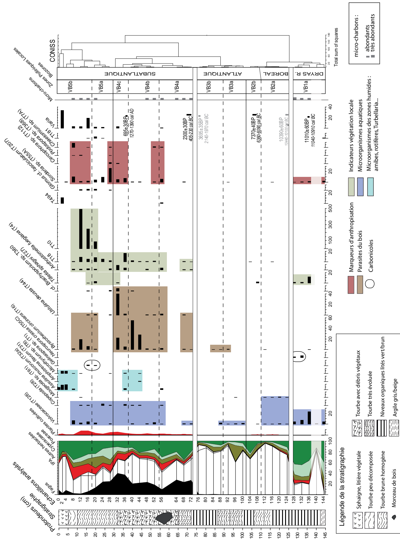
Fig. A.21. Tourbière du Verry-des-Brûlons - Diagramme des principaux Microfossiles Non-Polliniques (MNP)
