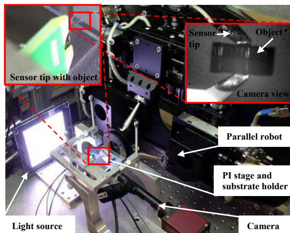
(b) Système expérimental de mesure
