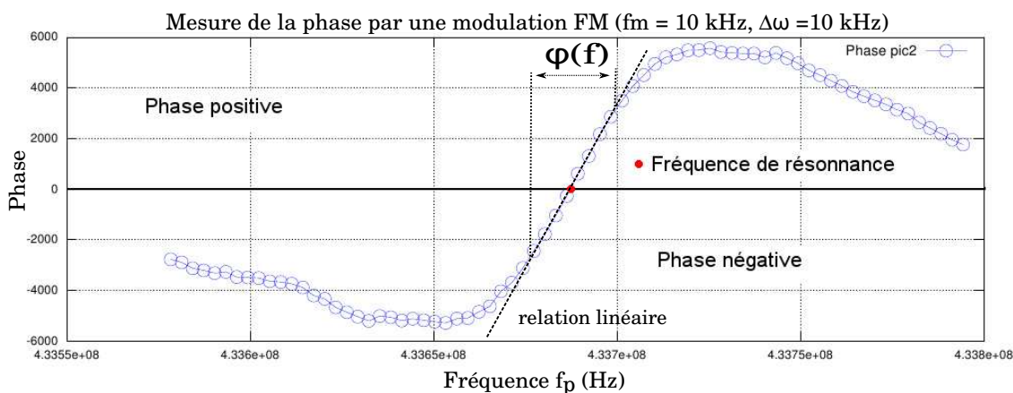
FIGURE 2.21 – Rotation de phase de chaque coté de la fréquence de résonance
