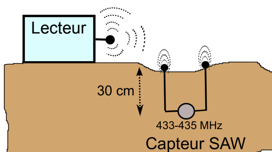
(a) Capteur de température enterré
