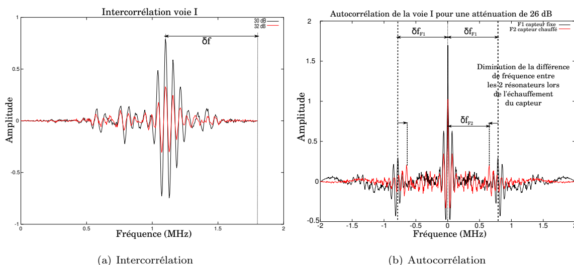
FIGURE 3.13 – (a) Intercorrélation des signaux de la première partie de la bande ISM avec la seconde partie. Le maximum d'intercorrélacion est situé à une abscisse proportionnelle à l'écart de fréquences entre les deux résonances, la mesure de \delta f permet obtenir cette écart de fréquence. (b) autocorrélation du signal contenant les deux résonances, les courbes F1 et F2 sont obtenues avant et après échauffement du capteur par une source de chaleur. L'écart de fréquence entre les deux résonances est donné par la moitié de la distance entre les deux lobes secondaires ( \delta f ) de part et d'autre du lobe principal correspondant au retard nul de l'autocorrélation.
