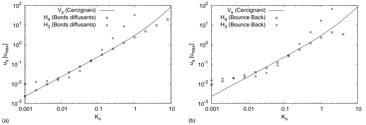
FIG. 3 – Vitesse de glissement en fonction du Knudsen pour les modèles basés sur \mathcal{H}_3 ( \circ ) et \mathcal{H}_4 ( \square ), avec des conditions aux bords diffusants (a) et des conditions aux bords de type Bounce-Back (b).
