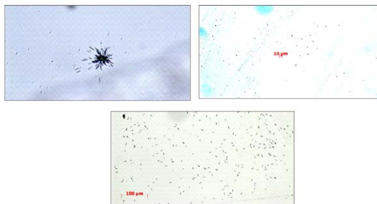
Рис. 4. Распределение треков на слюдяном детекторе от делирующих элементов в крови жителей г. Северска (верхний слева), г. Стржевского (верхний справа) в сравнении с распределением треков от урана-235 в контрольном образце (нижний). Увеличение указано линейкой на рисунках
