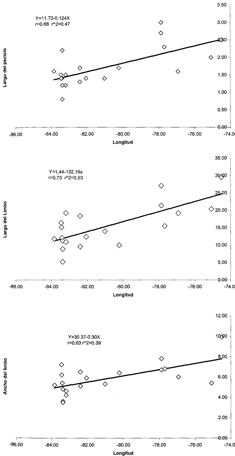
Fig.10. Regresión entre el largo y ancho del limbo, largo del peciolo y las longitudes geográficas en que se colectaron las muestras de Tetracera volubilis . y= a+bx ; a- 10. intersepto; b- pendiente; r- coeficiente de correlación.
