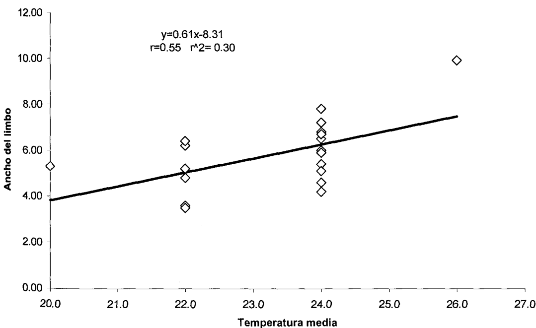
Fig. 12. Regresión efectuada entre el largo y ancho del limbo y la temperatura media anual en las localidades de colectas de los ejemplares de Tetracera volubilis . y= a+bx ; a- intersepto; b- pendiente; r- coeficiente de correlación.
