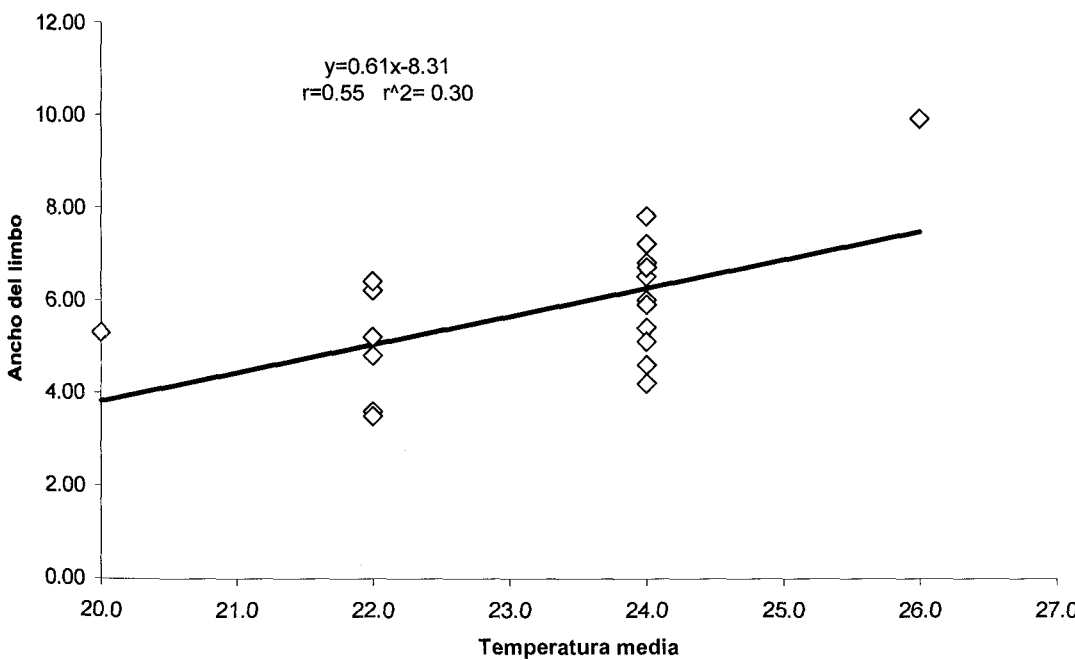
Fig. 12. Regresión efectuada entre el largo y ancho del limbo y la temperatura media anual en las localidades de colectas de los ejemplares de Tetracera volubilis . y=a+bx ; a- intersección; b- pendiente; r- coeficiente de correlación.
