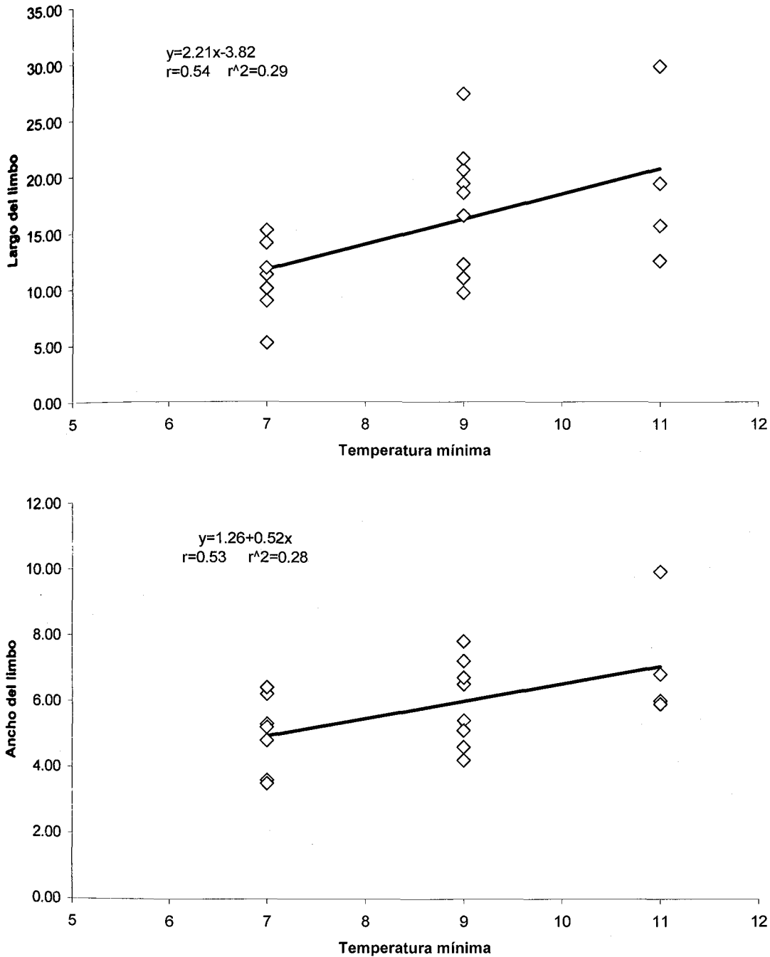
Fig. 13. Regresión efectuada entre el largo y ancho del limbo y la temperatura mínima absoluta en las localidades de colectas de los ejemplares de Tetracera volubilis . y=a+bx ; a- intersepto; b- pendiente; r- coeficiente de correlación.
