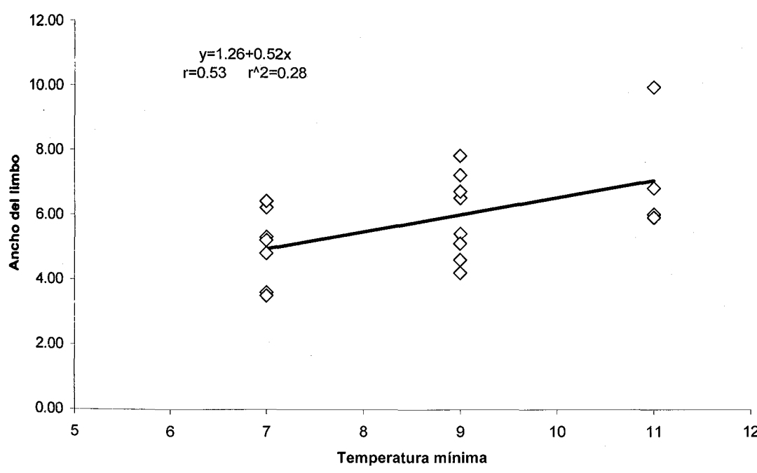
Fig. 13. Regresión efectuada entre el largo y ancho del limbo y la temperatura mínima absoluta en las localidades de colectas de los ejemplares de Tetracera volubilis . y=a+bx ; a- intersepto; b- pendiente; r- coeficiente de correlación.
