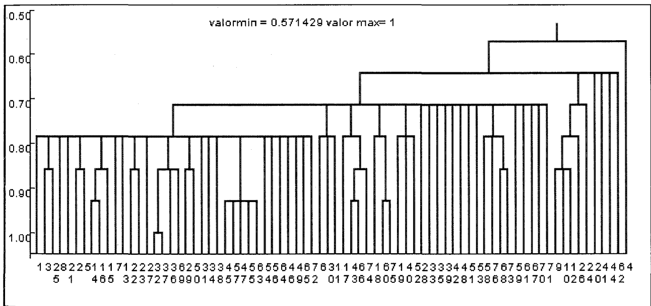
Fig. 5. Dendrograma obtenido por el método de Componentes Conexas para las muestras de Davilla .
