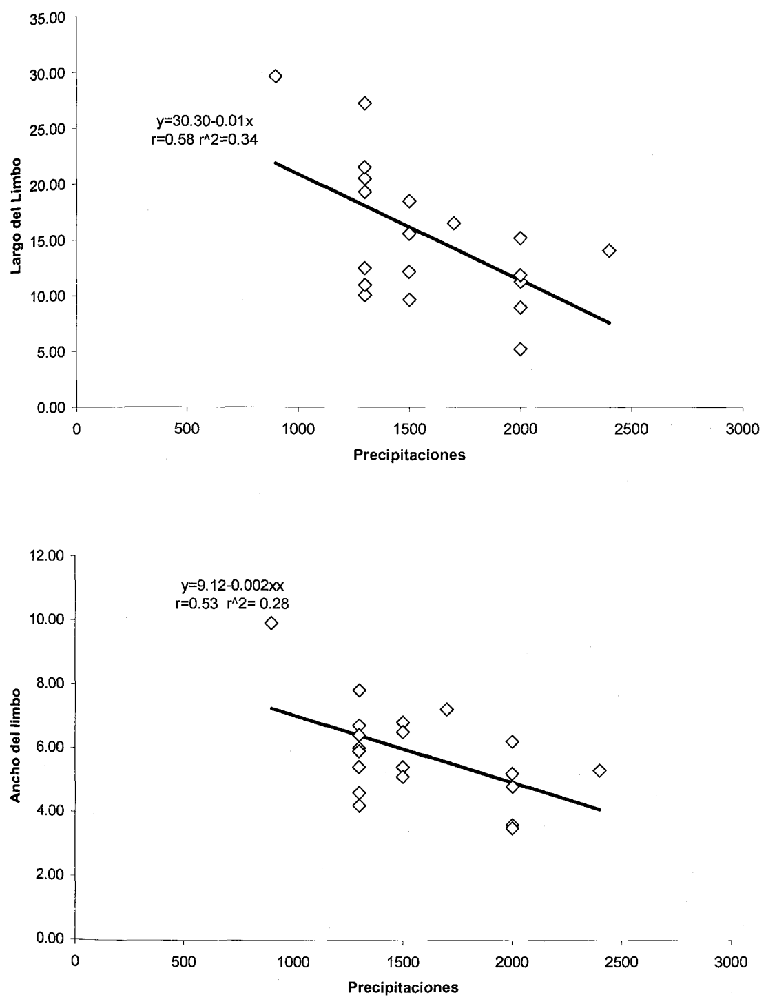
Fig. 11. Regresión efectuada entre el largo y ancho del limbo y la precipitación media anual en las localidades de colectas de los ejemplares de Tetracera volubilis . y=a+bx ; a- intersepto; b- pendiente; r- coeficiente de correlación.
