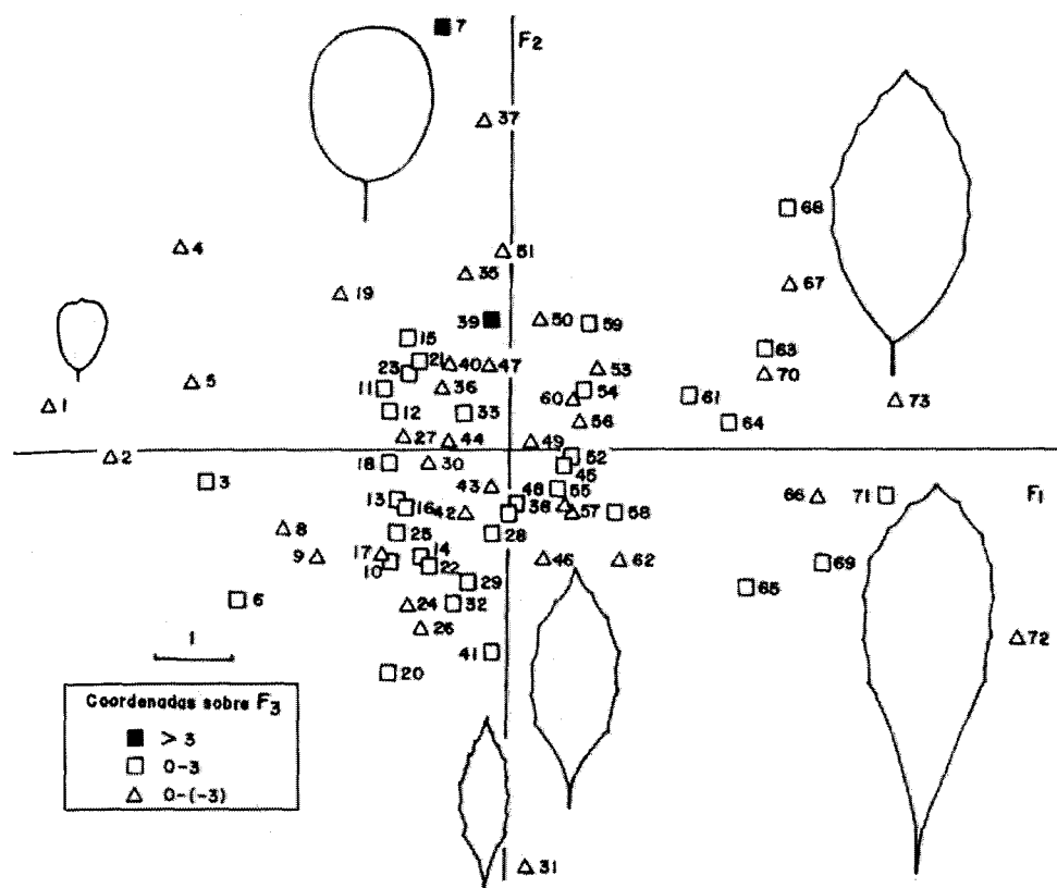
Fig. 4. Gráfico del Análisis de Componentes Principales para las muestras de Davilla nitida .
