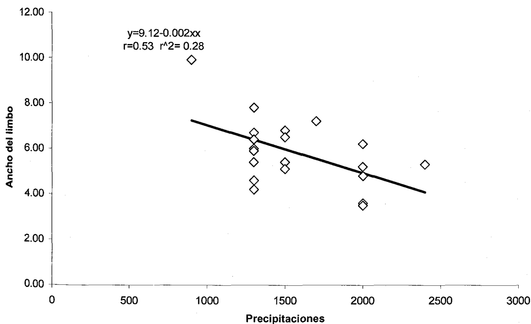
Fig. 11. Regresión efectuada entre el largo y ancho del limbo y la precipitación media anual en las localidades de colectas de los ejemplares de Tetracera volubilis . y=a+bx ; a- intersección; b- pendiente; r- coeficiente de correlación.
