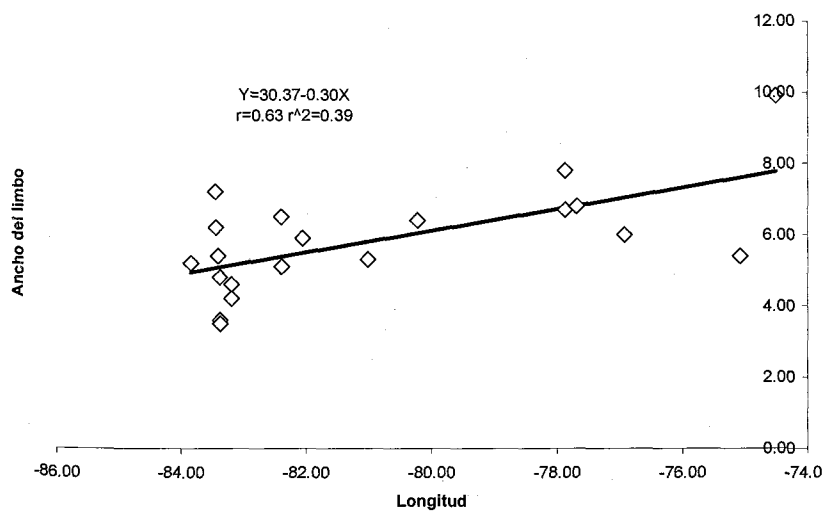
Fig.10. Regresión entre el largo y ancho del limbo, largo del peciolo y las longitudes geográficas en que se colectaron las muestras de Tetracera volubilis . y = a + bx ; a- 10. intersepto; b- pendiente; r- coeficiente de correlación.
