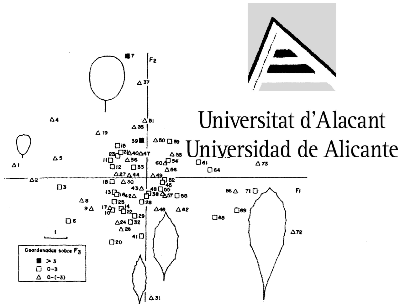
Fig. 4. Gráfico del Análisis de Componentes Principales para las muestras de Davilla nitida .
