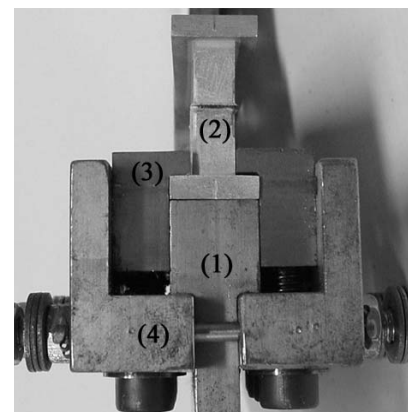
1 - support du montage Arcan 2 - substrats collés 3 - système de fixation 4 - support du système de fixation
