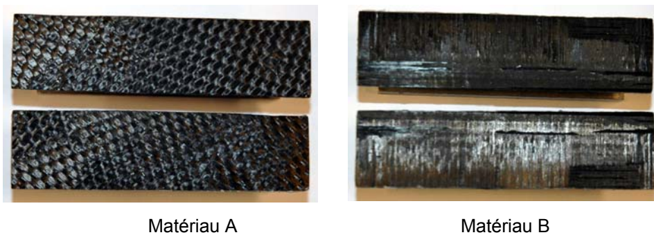
Fig 9 : faciès de rupture
