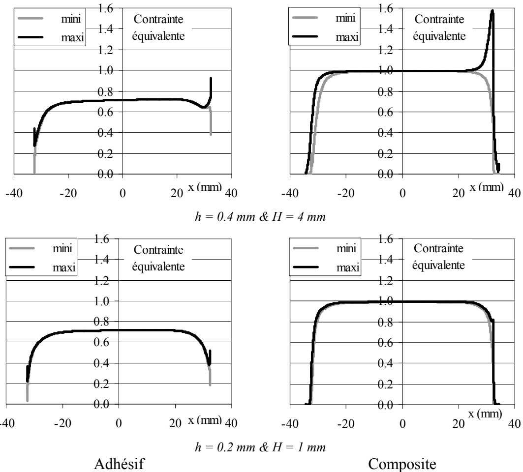
Fig 4 : Evolution de la contrainte équivalente de l'adhésif et du composite sous un chargement en traction-cisaillement (substrats avec bec ; stratifié avec D=2mm ).
