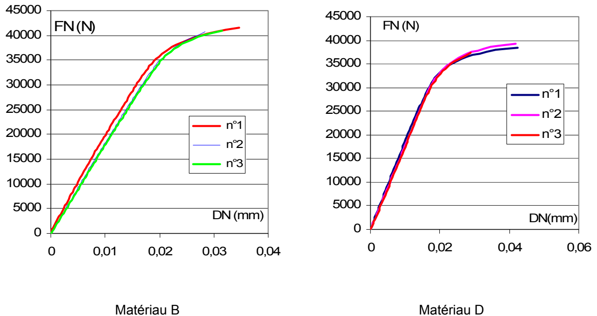
Fig 10 : analyse de différents composites
