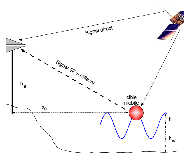
Figure 4.1 — Schéma de la cible sur la surface de mer
