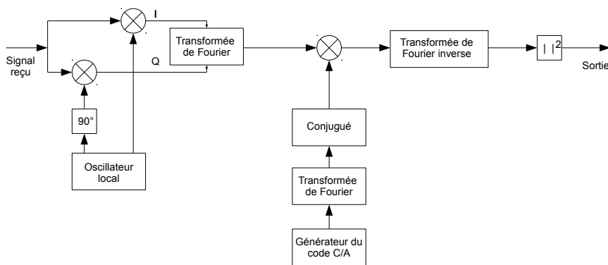
Figure 2.8 — Acquisition en mode parallèle du code et de la phase
