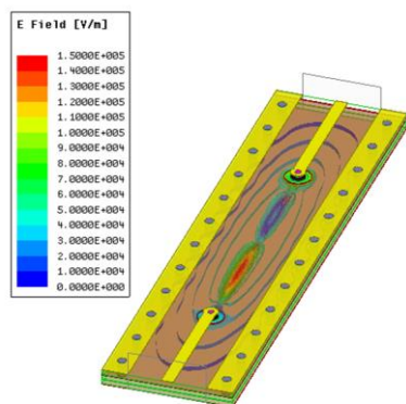
Figure 3: Lignes de champ électrique dans le substrat entre le plan M2 et M4 à 32 GHz.
