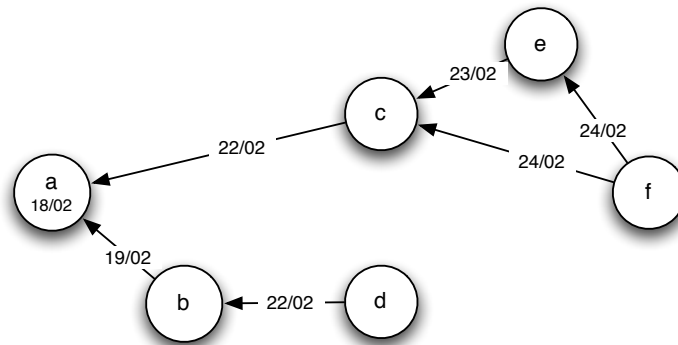
FIGURE 7.3: Illustration d'un sous-graphe de diffusion \sigma_{u_0} . Les étiquettes temporelles indiquent la date à laquelle les blogs ont simultanément mentionné u_0 et cité un blog de \mathcal{B} ayant déjà mentionné u_0 . NB : Les sous-graphes de diffusion ne forment pas nécessairement un arbre, comme en atteste le blog f sur cet exemple qui cite simultanément c et e comme sources.
