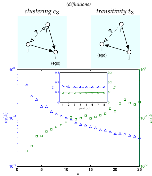
FIGURE 3.10: Coefficients de clustering c_3 (triangles bleus) et transitivity t_3 (carrés verts) en fonction du capital social k (encart : évolution des valeurs moyennes sur les 8 périodes).
