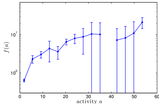
FIGURE 3.2: Attachement préférentiel en fonction de l'activité a , mesurée en nombre moyen de liens sortants créés hebdomadairement
