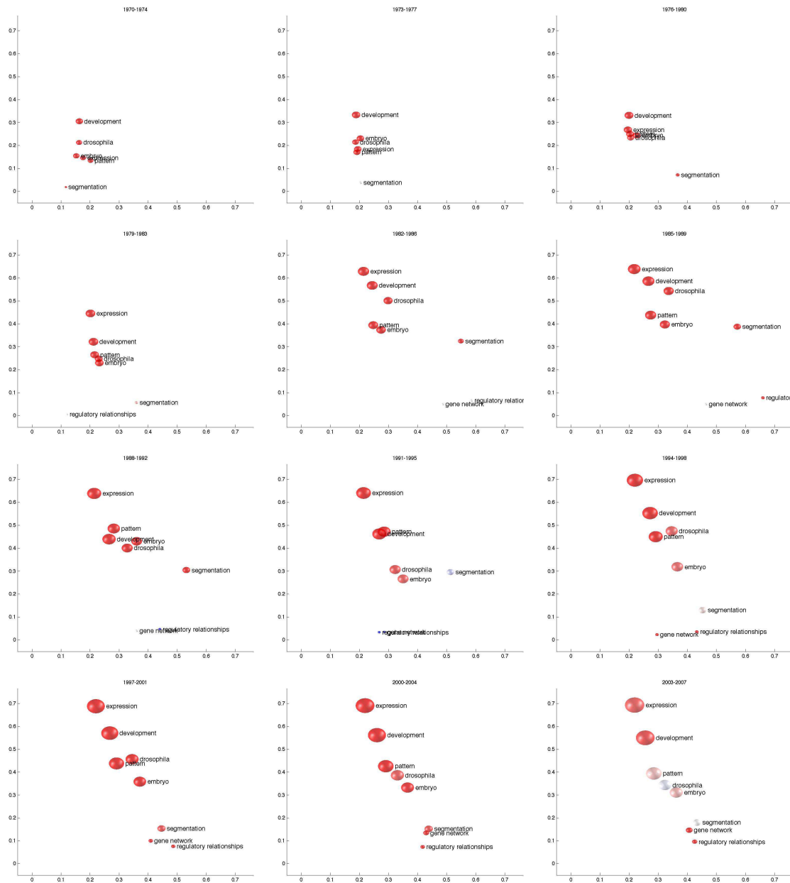
FIGURE 4.15: Evolution de la structure d'un champ épistémique détecté durant la période 2003-2007. Les années croient de gauche à droite et de haut en bas (depuis la période 1970-1974) par fenêtres glissante se décalant de 3 ans à chaque représentation. L'indice de spécificité I_s est en abscisse, l'indice de généricité en ordonnées I_g . La taille d'un terme correspond à son importance dans le champ, la couleur représente son taux de croissance
