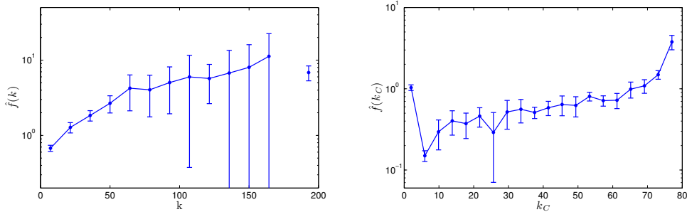
FIGURE 3.1: À gauche : propension d’interaction \hat{f} au degré social k . À droite : propension d’interaction \hat{f}_C au degré sémantique k_C . Moyenne sur 8 périodes. Afin de pallier le manque de données, celles-ci ont été regroupées dans des “bins” et tronquées dans le cas de l’attachement préférentiel au capital social ( k < 200 ).
