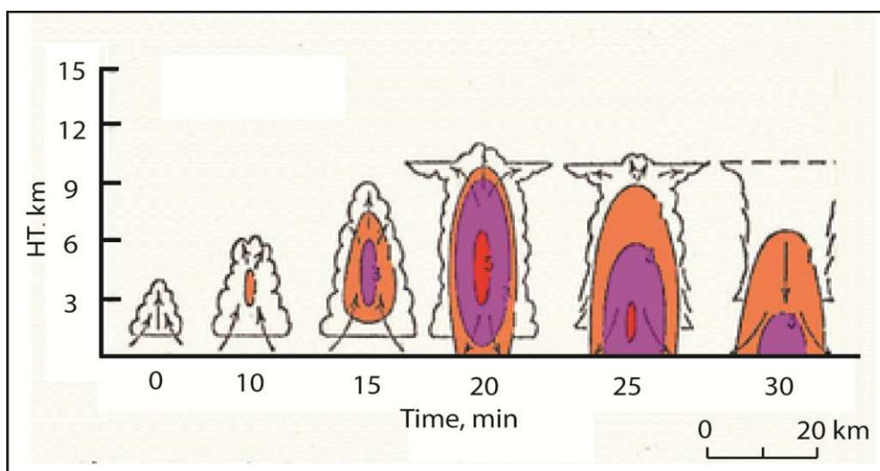
Fig. 4.5. Schéma d'un orage unicellulaire (adapté de Wilk et al. , 1977).
