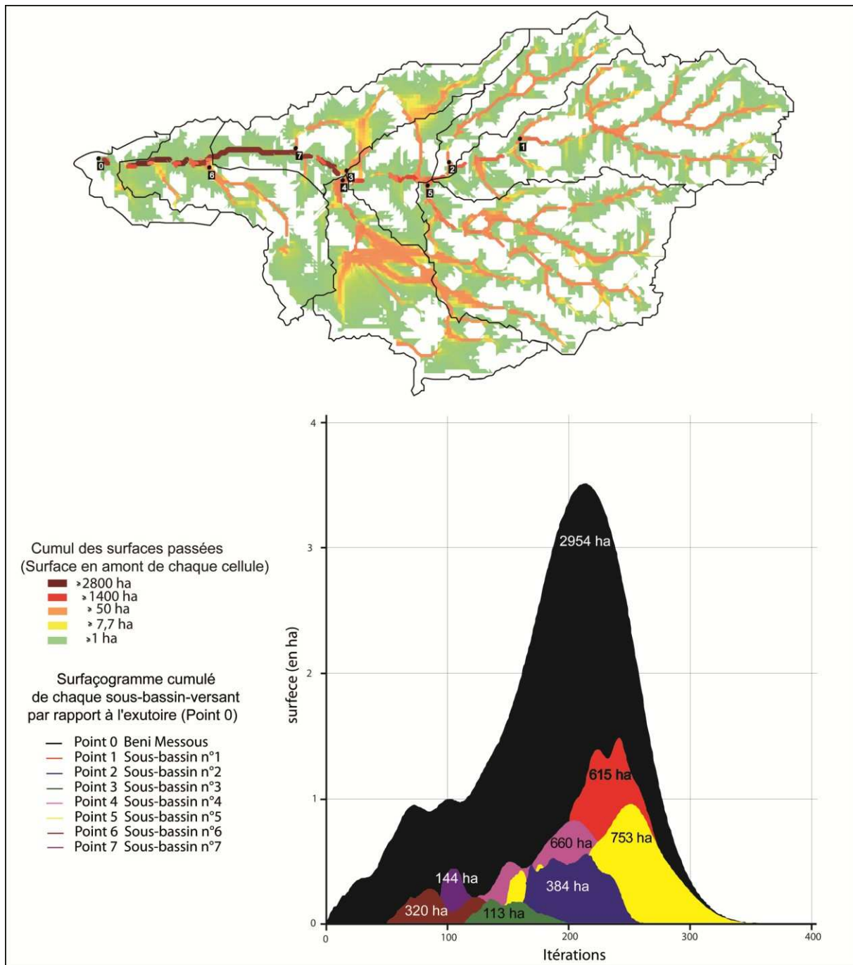
Fig. 6. 27. Simulation de la réponse hydrologique de Beni Messous dans l'espace 3D.
