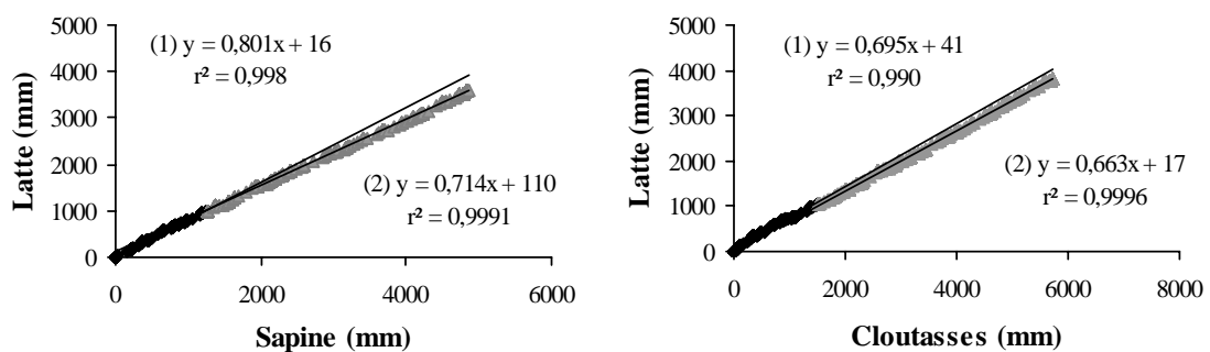
Fig. 3 Comparaison par double cumul des écoulements journaliers de crue du bassin de la Latte avec ceux des bassins de la Sapine et des Cloutasses de juillet 1981 à décembre 1998 (la période avant coupe est figurée en noir, celle après coupe en gris).
