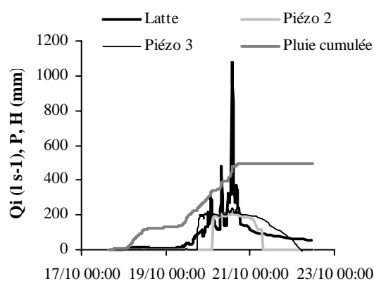
Fig. 5 Crue du 20 octobre 2001 sur le bassin versant de la Latte. Qi : débit instantané. P : précipitations. H : hauteur d'eau dans les piézograpes.
