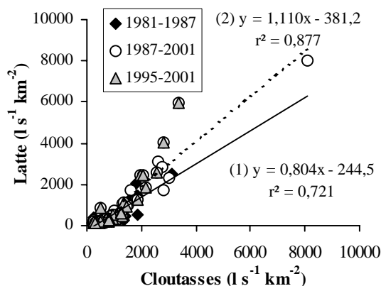
Fig. 4 Comparaison des débits spécifiques de pointe de crue maximaux mensuels des ruisseaux de la Latte et des Cloutasses sur la période août 1981 – décembre 2001.
