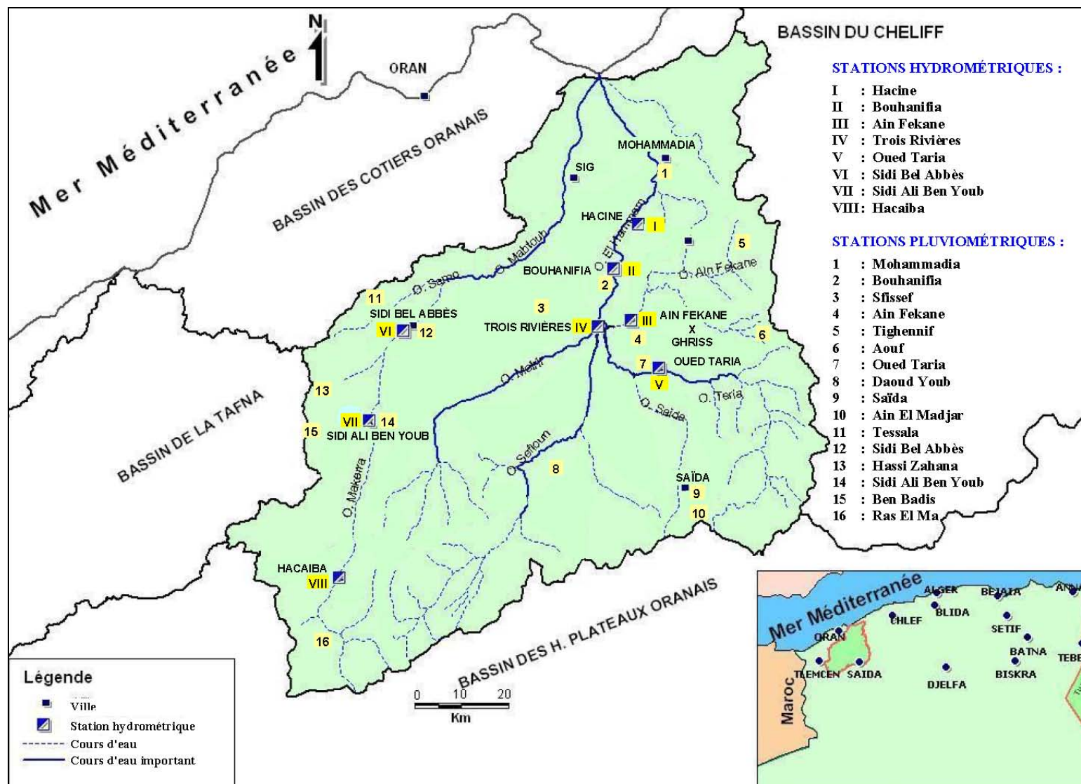
Figure 1 - Réseau hydrographique du bassin versant de la Macta.
