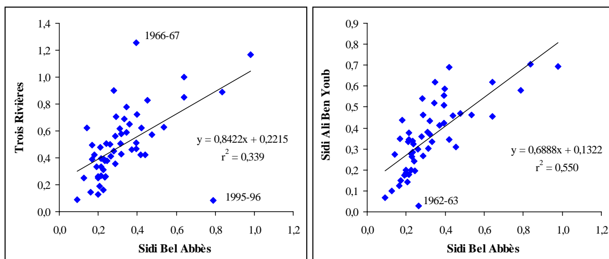
Figure 16 - Relations entre les débits spécifiques moyens annuels ( m^3/s/km^2 ) à la station de Sidi Bel Abbès et aux stations de Trois Rivières (1947-48 - 2001-02) et de Sidi Ali Ben Youb (1949-50 - 2001-02).
