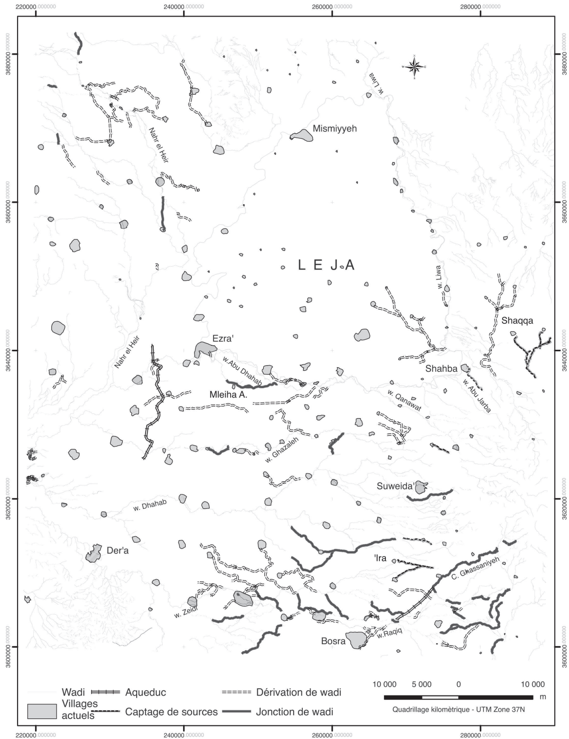
Fig. 17 - Carte des agglomérations et des aménagements hydrauliques du Hawran. Tous les villages installés le long des wādī possèdent une dérivation courte.
