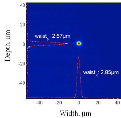
Fig. 2 : Observation en champ proche du mode d'un fil quantique @ \lambda = 1.5 \mu\text{m}
