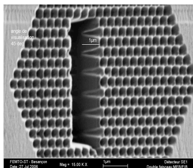
Fig. 1. Image au MEB d'un réseau de trous de 300nm de diamètre et de 1,5µm de profondeur, réalisés par FIB (FEMTO, Besançon) dans du niobate de lithium coupe X.
