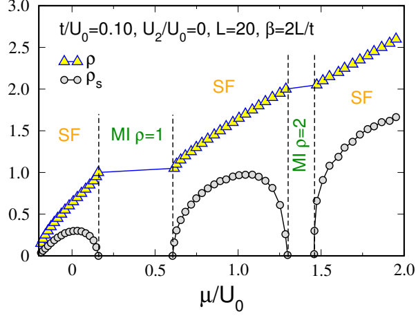
FIGURE 5.21 – Densité totale \rho et de la densité superfluide \rho_s en fonction du potentiel chimique \mu = E(N + 1) - E(N) pour U_2/U_0 = 0 avec L = 20 et \beta = 40/t . Ces courbes correspondent à la coupe verticale du diagramme de phase Figure 5.20 représentée en trait discontinu situé en t/U_0 = 0.10 avec \rho_0 = \rho_\Lambda = \rho/2 . Les phases isolantes de Mott (MI) sont clairement identifiées par les deux plateaux de densité \rho = \{1, 2\} avec une densité superfluide nulle \rho_s = 0 . La phase superfluide (SF) est compressible \partial\rho/\partial\mu \neq 0 avec une densité superfluide non nulle \rho_s \neq 0 . Aucune discontinuité n'est visible dans l'évolution de ces deux quantités: toutes les transitions sont du second ordre, en accord avec l'analyse en champ moyen.
