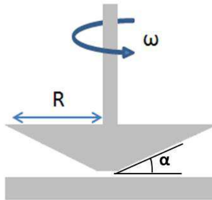
Figure VI.4 : Géométrie cône/plan
