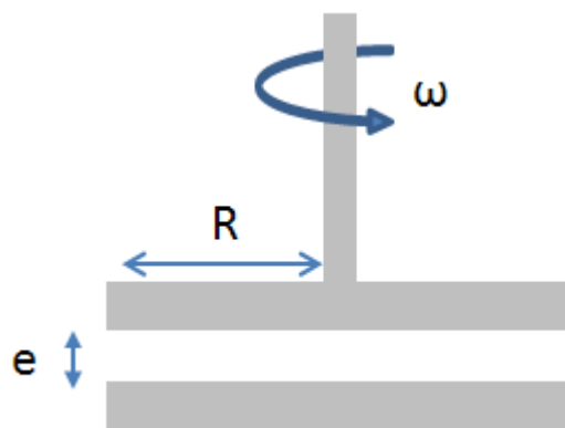
Figure VI.5 : Géométrie plan/plan
