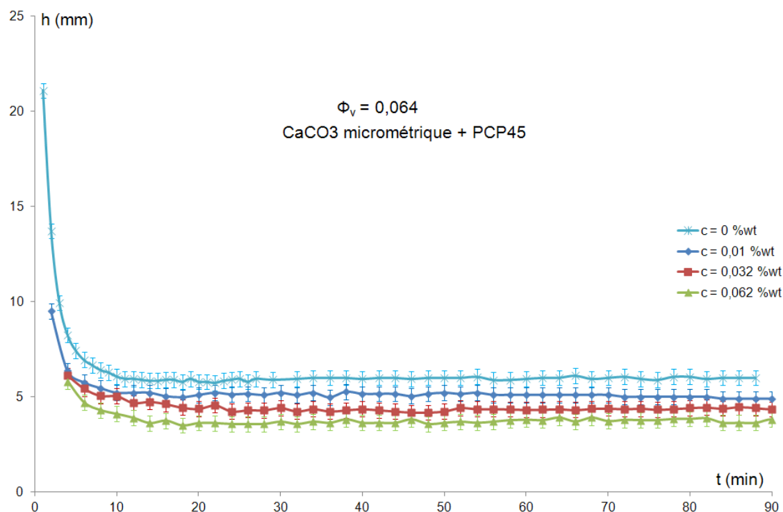
Figure V.3 : Hauteur du dépôt en fonction du temps pour des suspensions micrométriques adjugantées en PCP45
