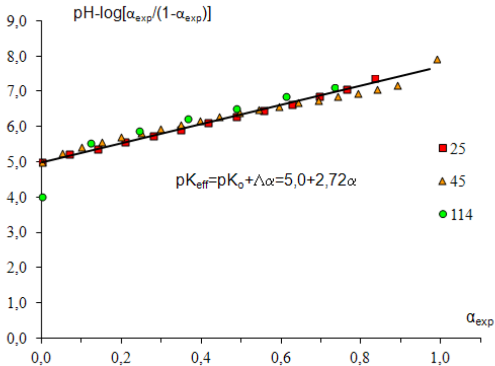
Figure III.14: pK_{\text{eff}} des différents PCP
