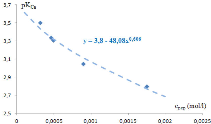
Figure III.22 : pK du calcium du PCP45 en fonction de la concentration en PCP
