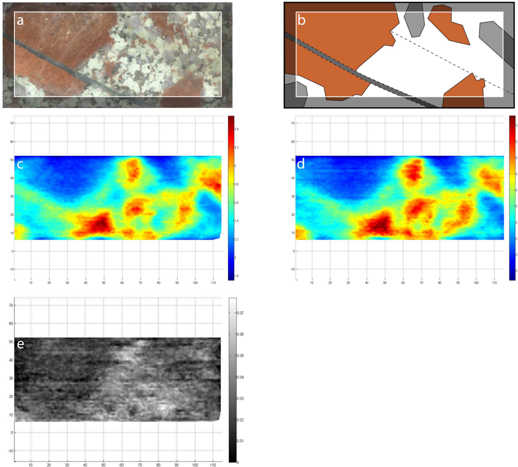
(a) photo de l'échantillon et délimitation de la zone scannée, (b) schéma minéralogique et structural, (c) carte de conductivité thermique de l'échantillon sec, (d) carte de conductivité thermique de l'échantillon saturé, (e) carte de densité de porosité.
