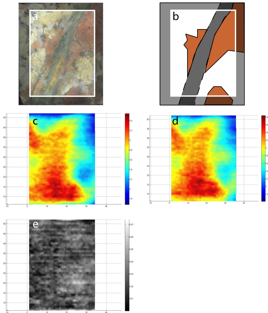
(a) photo de l'échantillon et délimitation de la zone scannée, (b) schéma minéralogique et structural, (c) carte de conductivité thermique de l'échantillon sec, (d) carte de conductivité thermique de l'échantillon saturé, (e) carte de densité de porosité.
