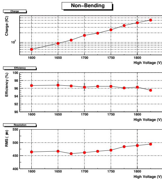
FIG. 3.47 – Charge des agrégats, efficacité à \pm 1\text{mm} , et résolution en fonction de la haute-tension dans le plan de non-courbure.
