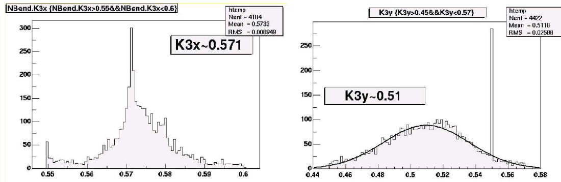
FIG. 3.54 – Résultat de l’ajustement des paramètres de Mathieson pour une prise de données des tests de la latte d’octobre 2001. Ajustement du paramètre K_{3x} sur la figure de gauche, et du paramètre K_{3y} sur la figure de droite. La valeur initiale de l’ajustement de K_{3x} et K_{3y} est 0.55 : des évènements rejetés apparaissent à ces valeurs.
