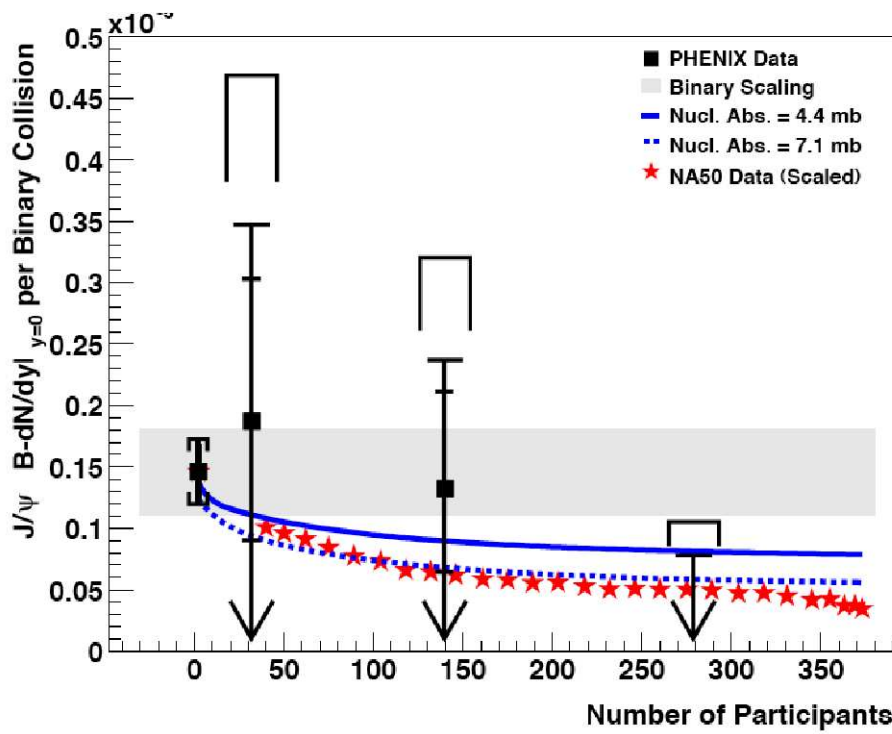
FIG. 1.24 – Production du J/\psi par collision binaire en fonction du nombre de participants (carrés pleins) lors de collisions à \sqrt{s_{NN}} = 200 \text{ GeV/nucleon} , mesurée par l'expérience PHENIX. Pour comparaison, les données de l'expérience NA50 (étoiles) sont rapportées à la production de J/\psi en collision p-p [45].
