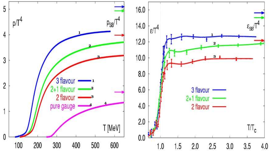
FIG. 1.2 – Rapports p/T^4 en fonction de T (figure de gauche) et \epsilon/T^4 en fonction de \frac{T}{T_c} (figure de droite) issus d'un calcul sur réseau avec différentes valeurs de quarks. \epsilon_{SB} est la densité d'énergie de Stefan-Boltzmann. Ces calculs sont détaillés [37].
