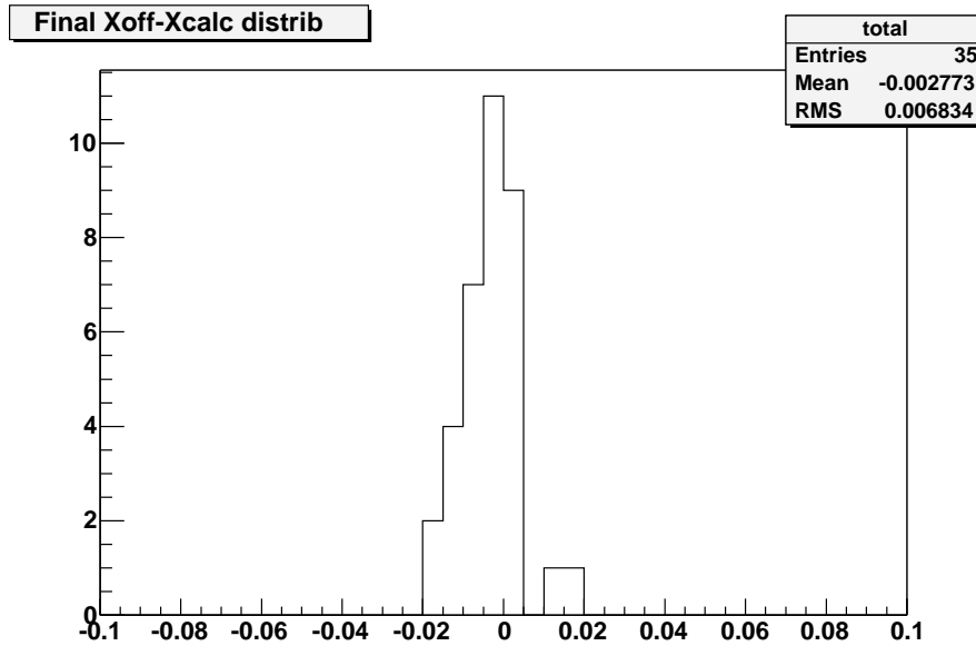
FIG. 4.22 – Distribution X_{\text{rél}}-X_{\text{calculé}} (en cm) de l'ensemble des lattes touchées, résultant de l'alignement avec champ magnétique.
