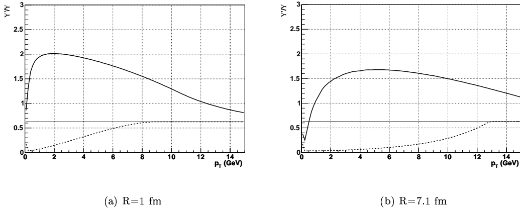
FIG. 5.8 – Rapport de production directe (prompte) \left[\frac{\Upsilon'}{\Upsilon}\right]^d en fonction du moment transverse dans les cas PQG-SU(N) (trait plein), et PQG-SU(3) (pointillés) pour deux choix de rayons.
