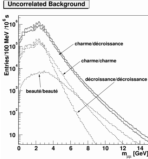
FIG. 5.17 – Spectre en masse invariante \mu^+\mu^- du bruit de fond non-corrélé reconstruit avec le spectromètre dimuon de l'expérience ALICE et correspondant à une prise de données de 10^6 s et pour des intervalles de 100 \text{ MeV}/c^2 : les contributions beauté/beauté (alternés), décroissance/décroissance (pointillés), charme/charme (tirets) et charme/décroissance (trait fin) sont sommées (trait épais). Une coupure de 1 \text{ GeV}/c a été utilisée sur l'impulsion transverse des muons individuels.
