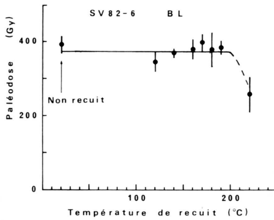
Fig. 6. — Test de plateau pour les paléodoses obtenues avec BL, après des recuits à des températures différentes.
