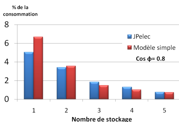
Figure 61- Réduction de perte Joule du cas \cos\phi=0.8
