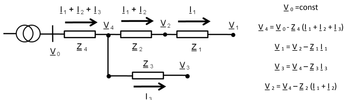
Figure 69 – Calcul de répartition BFS (backward-forward sweep)
