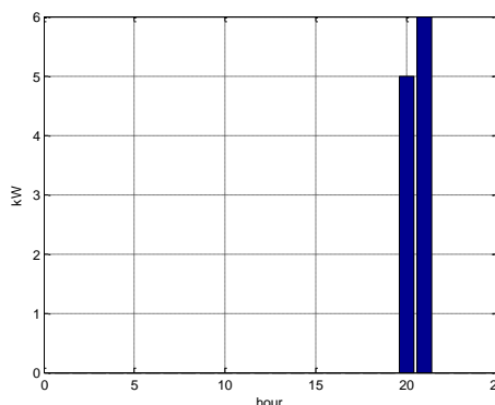
Figure 58- Profil de production de groupe électrogène n° 1.
