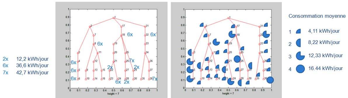
Figure 70 –Répartition de production PV et de consommation
