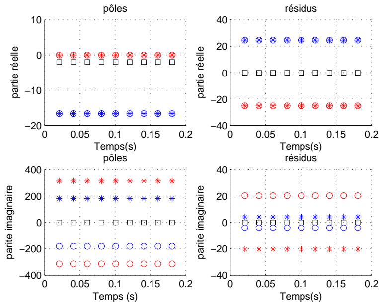
FIGURE 3.26 – Suivi temporel des pôles et résidus normalisés dans le cas l'enclenchement simultané d'une charge R_1C_1 série mise en parallèle avec une charge R_2L_2C_2 série R_1 = 10 \Omega , C_1 = 50 \text{ mF} et R_2 = 1 \Omega , C_2 = 30 \text{ mF} , L_2 = 1 \text{ mH}
