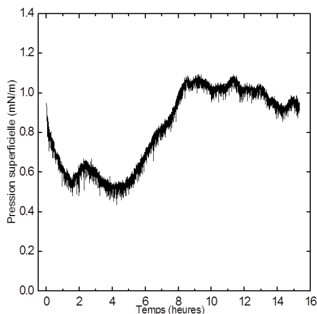
Figure 7.10: Stabilité temporelle d'une monocouche de PS-b-PAA non éclairée, initialement comprimée à \Pi = 0.8 mN/m sur une sous-phase à \text{pH} = 9 + (\text{Ag}^+) et à T = 18 °C.
