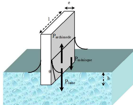
Figure 4.2: Principe de mesure de la pression superficielle avec une lame de Wilhelmy.
