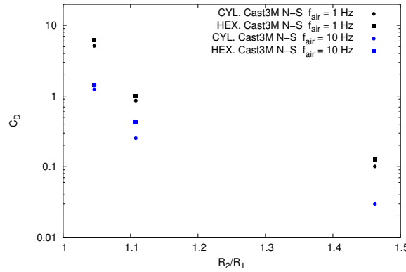
FIGURE 5.25 – Effets de la géométrie : comparaison des valeurs des coefficients C_M et C_D obtenues par les modèles « Cast3M Navier-Stokes » et up\phi pour deux hexagones concentriques et deux cylindres concentriques
