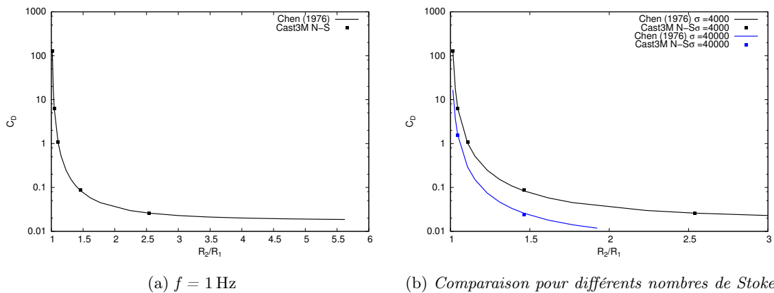
FIGURE 5.4 – Comparaison du coefficient d'amortissement en fonction du confinement dans le cas de deux cylindres concentriques
