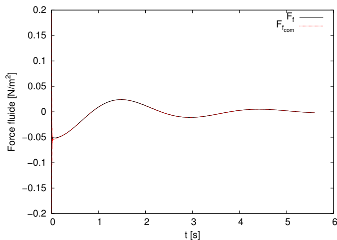
FIGURE 5.18 – Comparaison de la force fluide trouvé par « Cast3M Navier-Stokes » et par la formulation associée à C_M et C_D
