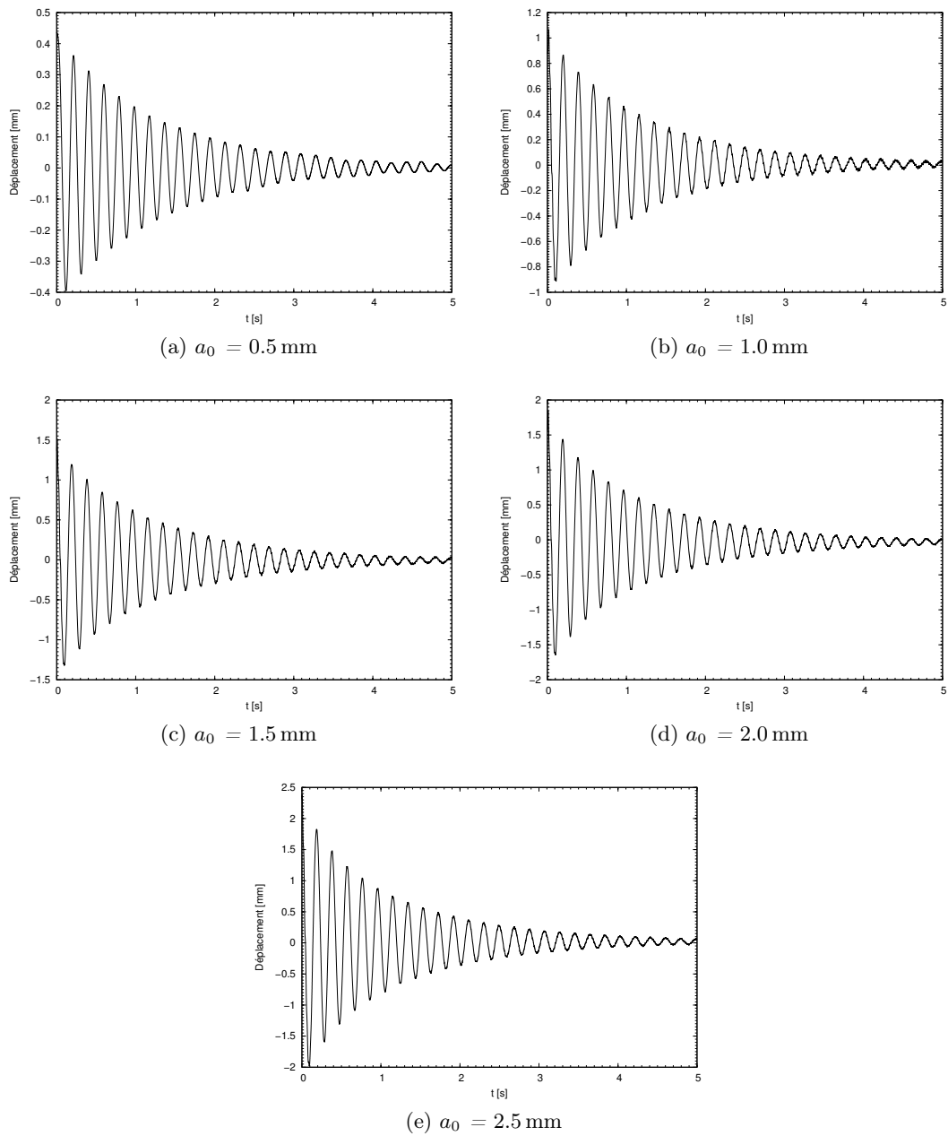
FIGURE 6.15 – Évolution dans le temps du déplacement de l'assemblage de PISE-1a lors des vibrations libres en eau mesuré avec un jauge de déformations pour différents déplacements initiaux a_0
