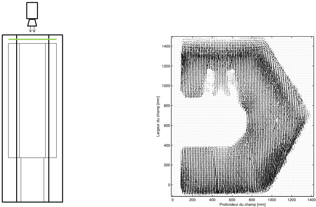
(a) Schéma du plan laser visualisé : dessus de la tête de l'hexagone
