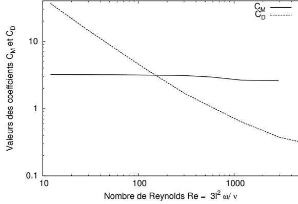
FIGURE 2.6 – Coefficient de masse ajoutée C_M et d’amortissement ajouté C_D pour deux hexagones concentriques [49]
