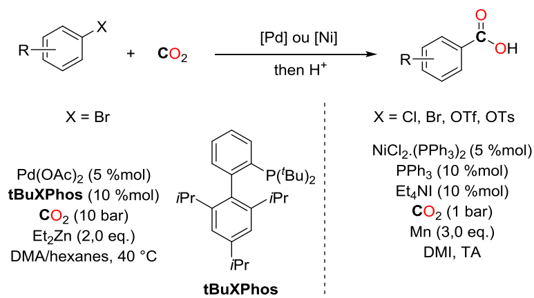
Schéma 65 - Carboxylation de dérivés halogénés aromatiques
