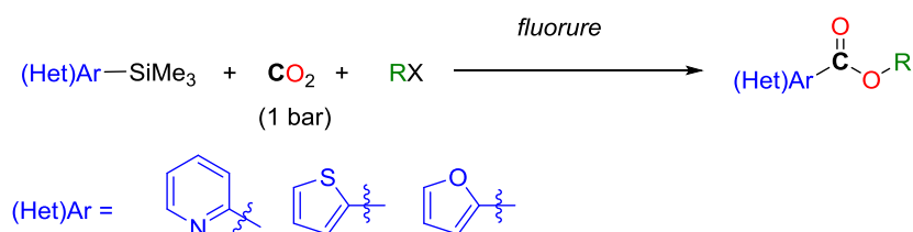
Schéma 130 - Carboxylation d'organosilanes en présence de fluorure
