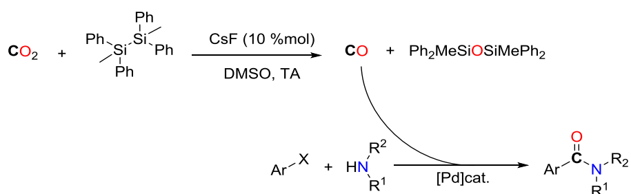
Schéma 80 - Couplage carbonyle à partir du CO 2
