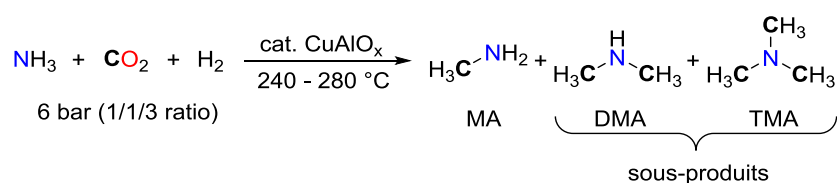
Schéma 19 - Méthylation de l'ammoniac par \text{CO}_2 et \text{H}_2
