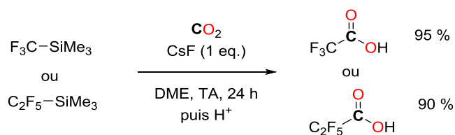
Schéma 83 - Synthèse de l'acide trifluoroacétique et pentafluoropropionique avec le CO 2
