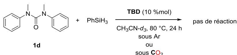
Schéma 54 - Tentative d'hydrosilylation organocatalysée de 1d
