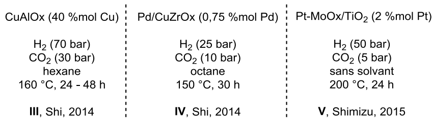
Schéma 44 - Systèmes catalytiques d'hydrogénation du CO 2 pour la méthylation des amines
