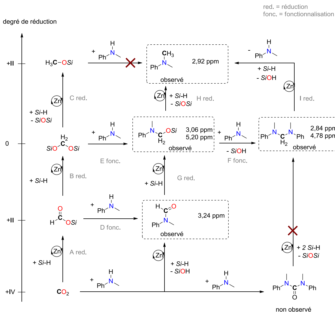
Schéma 41 - Voies réactionnelles plausibles
