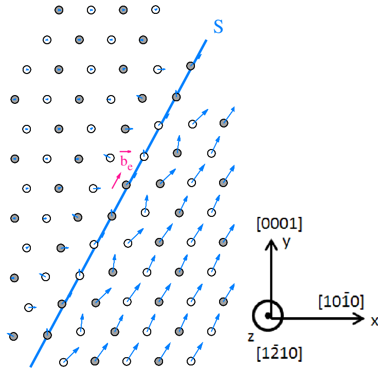
FIGURE 3.6 – Projection de la faute métastable pyramidale dans le plan (\bar{1}\bar{2}10) . Les flèches bleues sont proportionnelles aux déplacements des atomes parallèlement au plan (\bar{1}\bar{2}10) . Les ronds gris et blancs indiquent la positions des atomes le long de la direction [\bar{1}\bar{2}10] . La ligne continue bleue indique le plan initial de cisaillement de la faute S . Le vecteur \vec{b}_e est amplifié 3 fois.
