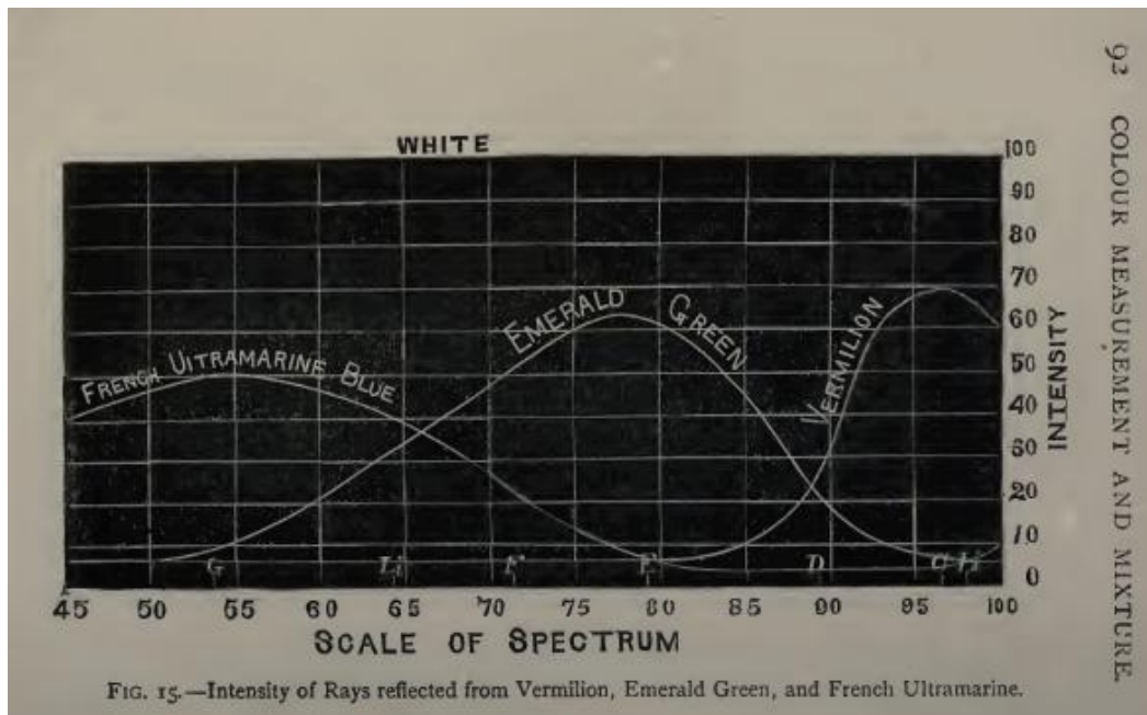
Figure I-14 Spectres d'intensité de trois pigments (Vermillon, Vert Émeraude et Outremer Français) par Abney (tiré de [Abney 1891], page 92)
