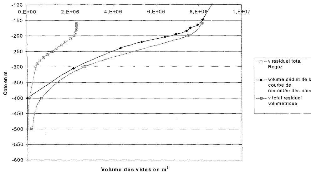
Figure 4. Comparaison entre la répartition selon la profondeur des volumes des vides résiduels cumulé par la méthode empirique de M. Rogoz (1978), par la méthode volumétrique et par le volume mesuré d'après la remontée de l'eau.
