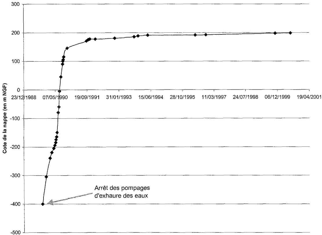
Figure 2. Courbe piézométrique de la remontée de la nappe souterraine au puits 1 de Faulquemont (HBL, 1999)
