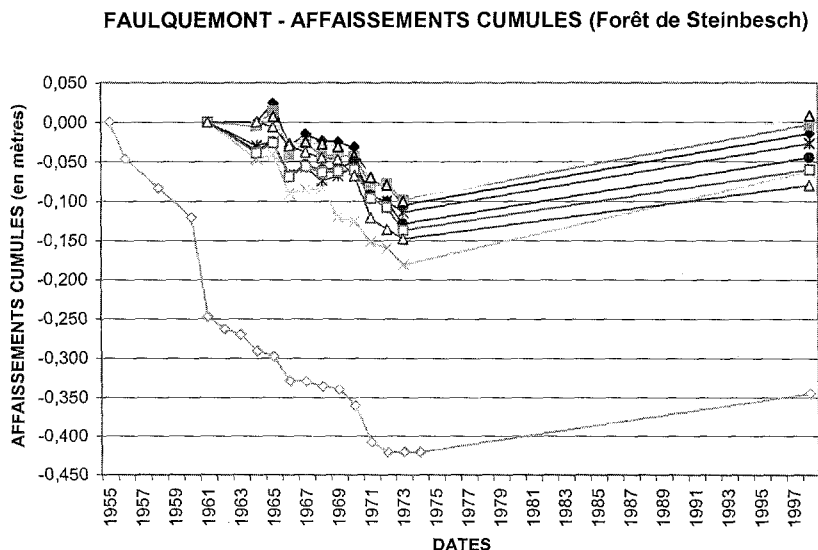
Figure 3. Mesures topographiques dans le secteur de Faulquemont (forêt de Steinbesch) après l'ennoyage des travaux.
