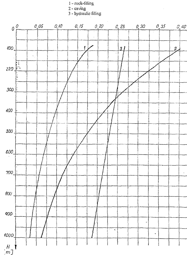
Figure 1. Détermination du coefficient de capacité à l'eau en fonction de la profondeur H (mètres) et du mode de traitement de l'arrière-taille (M. Rogoz, 1978)
