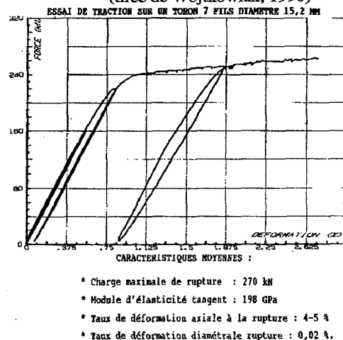
Figure 5: Propriétés mécaniques des câbles (tirée de Wojtkowiak, 1990)
