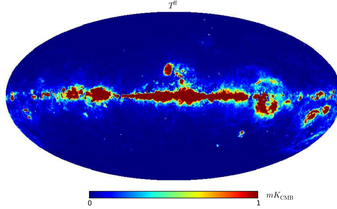
FIGURE 3.4 – Carte de l'émission libre-libre à 23 GHz extraite des données WMAP 3 ans par la méthode MEM (Hinshaw et al. , 2007). Cette carte est utilisée par les modèles mamd_dickinson_4comp et mamd2008 . Sa résolution est d'environ 1^\circ . L'ajout de petites fluctuations à cette carte utilise les valeurs \gamma = -2.6 , \alpha = 0.1 , \beta = 1.1
