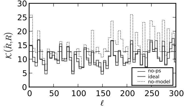
FIGURE 5.5 – Ajustement pour les 3 cas décrits plus haut. Le cas de référence 'no-ps' n'inclut de sources ponctuelles, ni dans les données, ni dans le modèle d'ajustement. Le critère d'ajustement varie autour de sa valeur attendue (ligne horizontale pointillée). Le cas 'no-model' est un cas pessimiste, où aucun effort de modélisation n'est réalisé pour tenir compte de la contribution des sources ponctuelles. Dans ce cas, l'ajustement subit une nette dégradation. Le cas 'ideal' représente une situation idéale dans laquelle la contribution des sources ponctuelles incluses dans les simulations, est modélisée exactement, et qui permet de retrouver une qualité d'ajustement comparable au cas 'no-ps'.
