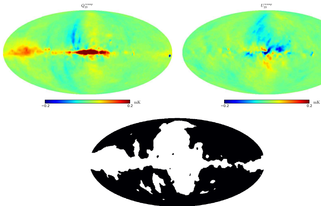
FIGURE 3.6 – Mesure de l'émission polarisée du ciel à 23 GHz par la sonde WMAP. La zone blanche sur le masque correspond à une mesure de la polarisation avec un niveau de signal sur bruit supérieur à 3.
