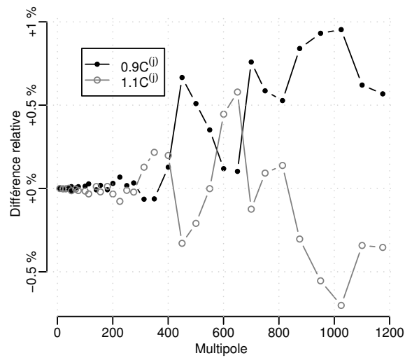
FIGURE 4.8 – Robustesse de l’estimateur spectral en needlets par rapport à la valeur a priori du spectre \overline{C}^{(j)} .
