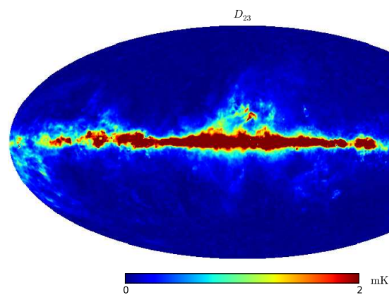
FIGURE 3.7 – Émission anormale de la poussière à 23 GHz extraite du modèle 4 proposé par Miville-Deschênes et al. (2008).
