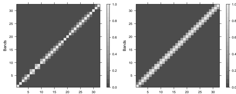
FIGURE 4.10 – Valeur absolue de la matrice de corrélation du vecteur (\widehat{C}^{(1)}, \dots, \widehat{C}^{(32)}) , pour deux familles de needlets (PSWF à gauche et Top-Hat à droite). La matrice est obtenue par la réalisation de 400 simulations Monte-Carlo du modèle décrit en figure 4.4.
