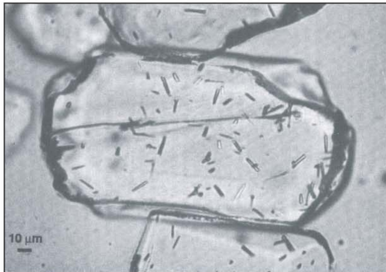
Photo 3.15 - Fissure subhorizontale et population de traces de fission dans un cristal hexagonal d'apatite (cliché aimablement communiqué par Gianni Gunnell).
