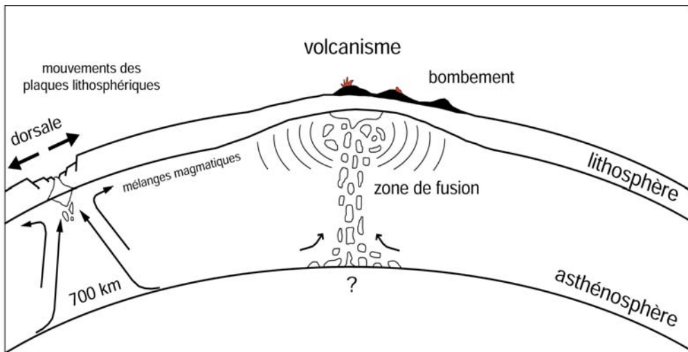
Fig. 1 – Croquis simplifié d'un panache mantellique. Des doutes subsistent quant à l'origine des remontées mantelliques, les interactions avec les mécanismes d'accrétion océanique et de subduction, et le rôle des points chauds dans la dynamique interne du globe terrestre.
