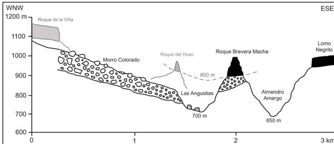
Fig. 2.26 - Coupe nord-ouest / sud-est du centre de la Caldera de Taburiente. Les coulées et matériaux volcanoclastiques Los Roques du Bejenado fossilisent l'ancien tracé du Barranco de las Angustias (850 m). Les dépôts d'un effondrement des parois ouest de la caldera (Risco de la Pared) affleurent sous les Roques.
