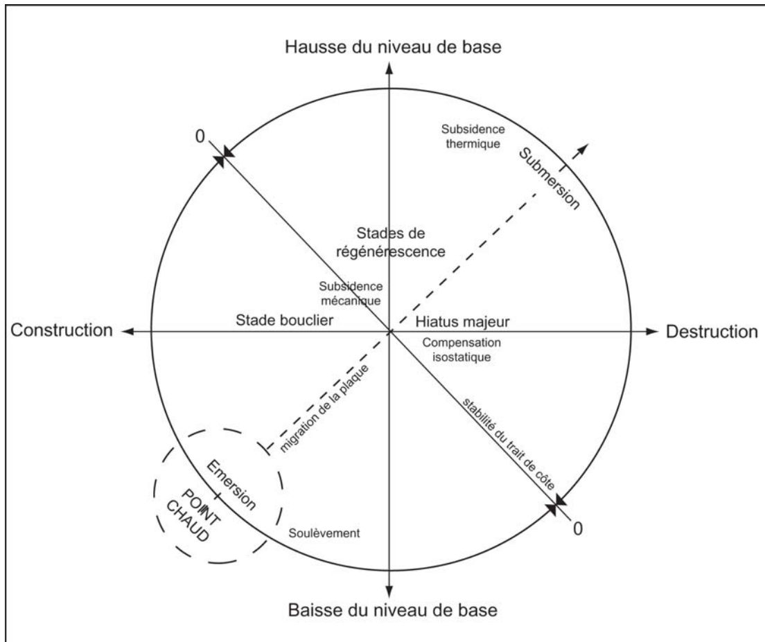
Fig. 3.33 - Les relations entre la construction, la destruction et les variations verticales du niveau de base d'une île de point chaud, d'après le modèle classique d'évolution des Iles Hawaiï ou Société. Ce schéma n'est plus valable aux Iles Canaries, du fait de la proximité de la marge continentale et de la lenteur de déplacement de la plaque africaine. Aucune phase de subsidence sur le long-terme n'est attestée aux Iles Canaries.
