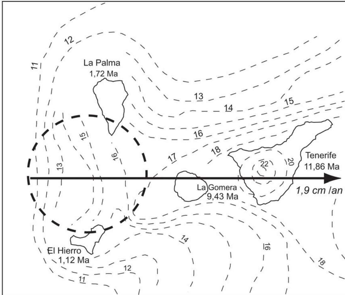
Fig. 1.9 - Dédoublément de l'alignement insulaire des Canaries en une ligne double La Palma - El Hierro : résultat des interactions entre l'affaissement flexural de la lithosphère sous Tenerife et La Gomera, le point chaud situé entre La Palma et El Hierro (cercle en tireté), et la faible mobilité de la plaque africaine (flèche). Les isocourbes représentent la profondeur du Moho en kilomètres, d'après les travaux de Bosshard & McFarlane (1970, Journal of Geophysical Research 75-26 p 4903).
