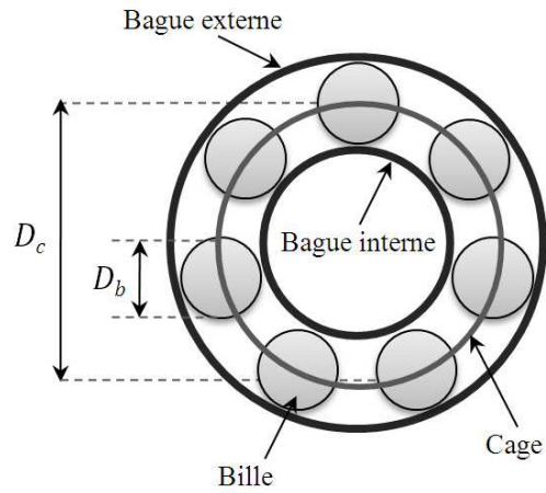
FIGURE 1.3: Structure d'un roulement à billes
