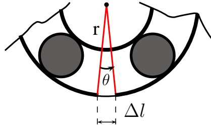
FIGURE 2.3: Modélisation du défaut de course externe
