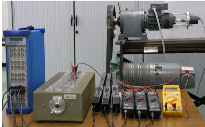
FIGURE 1.4: Banc d'essai
