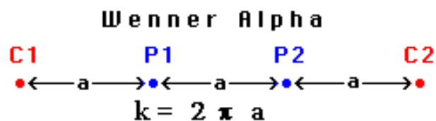
Figure III-28 : Position des électrodes d'injection du courant (C) et des électrodes de potentiel (P) avec un protocole Wenner- \alpha . Le facteur géométrique k , propre à chaque configuration, entre dans le calcul de la résistivité apparente ; a est l'écartement entre les électrodes, ici identique entre chaque électrode activée.
