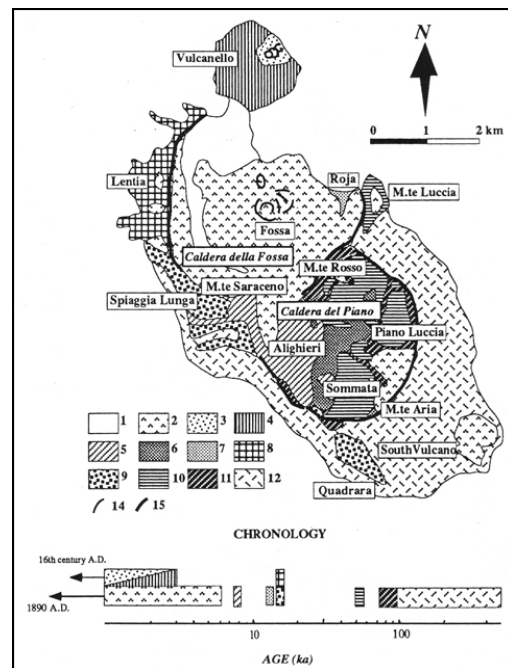
Figure II-17 : Géologie simplifiée et chronologie de Vulcano (dans Ventura, 1994 d'après Keller, 1980 et De Astis et al., 1989). 1 : alluvions ; 2 : produits de la Fossa ; 3, 4 : Vulcanello ; 5 : pyroclastites (Alighieri) et laves (Saraceno) ; 6 : cendres ; 7 : laves de Roja ; 8 : Lentia ; 9, 10, 11, 12 : pyroclastites et laves ; 11 : produits anciens de remplissage de la caldera du Piano ; 13 : cratères ; 14 : limites des calderas
