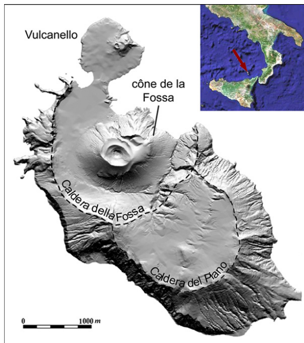
Figure II-16 : L'île de Vulcano (Italie, Iles Eoliennes). Sur cette île, deux calderas marquent le paysage. La plus récente, la caldera en fer à cheval de la Fossa, est ouverte sur la mer en direction du Nord-Est (modifiée d'après Ferrucci et al. 2005)
