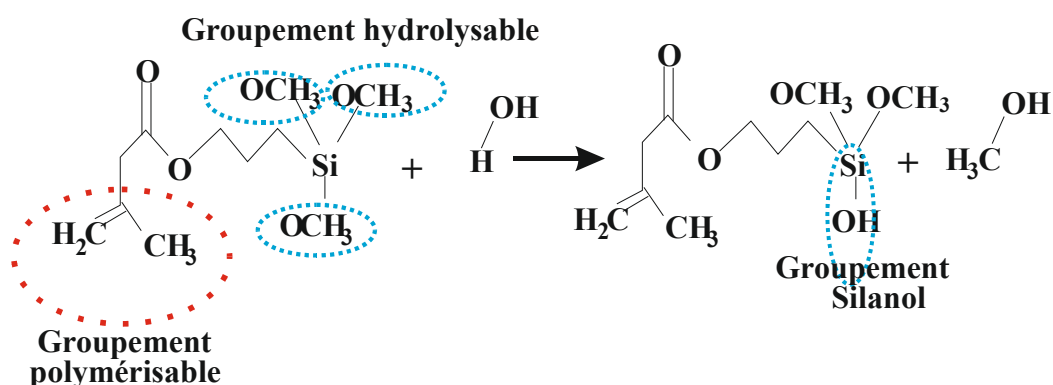
Figure II- 18: Pré-hydrolyse du méthacryloxypropyltriméthoxysilane (MAPTMS).
