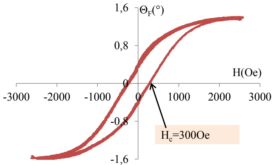
Figure III- 16: La conversion de mode magnéto-optique dans la structure hybride ( \lambda = 1550 \text{ nm} ).
