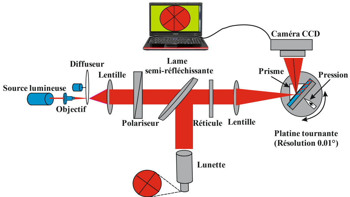
Figure II- 26 : Banc de mesure de spectroscopie de lignes noires. Un faisceau convergent de lumière éclaire le prisme. Il y a couplage ce qui apparaît comme une ligne noir sur l'écran.
