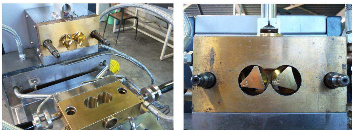
Figure 82 : Mélangeur interne Rheomix Thermo Haake 600 équipé de pâles roller rotor, disponible à l'IMP@UJM 1
