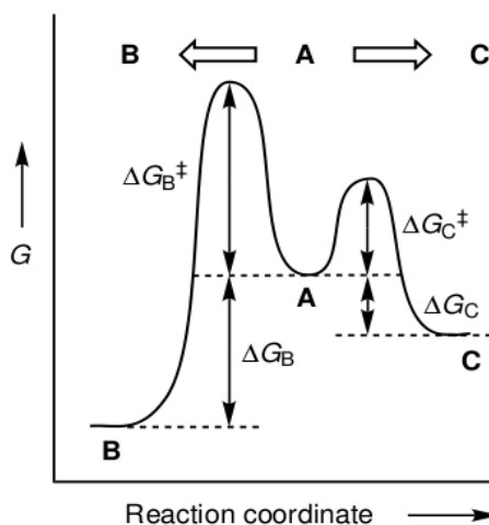
Figure 21 : Profil de l'énergie libre illustrant les contrôles cinétiques ( A \rightarrow C ) et thermodynamiques ( A \rightarrow B ) de la distribution de produits 68
