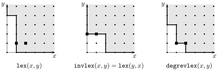
FIGURE 9.7 – Escaliers de l'idéal \langle xy + x + y^2 + 1, x^2y + xy^2 + 1 \rangle \subset \mathbb{Q}[x, y] relativement à différents ordres monomiaux.
