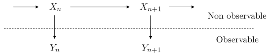
FIG. 6.1 – Diagramme de dépendance pour un modèle de Markov caché. Conditionnellement à X_{0:n} et Y_{0:n} , la loi de X_{n+1} ne dépend que de X_n . De même, conditionnellement à X_{0:n+1} et Y_{0:n} , la loi de Y_{n+1} ne dépend que de X_{n+1} .
