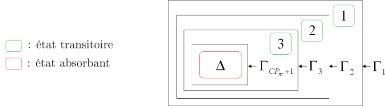
FIG. 3.3 – Représentation des ensembles \Gamma_k pour CP_m = 3 .
