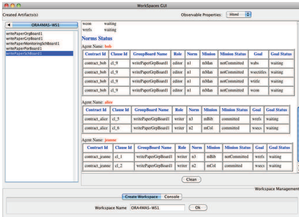
(b) Propriétés observables "NormStatus" pour les agents bob, alice et jeanne
