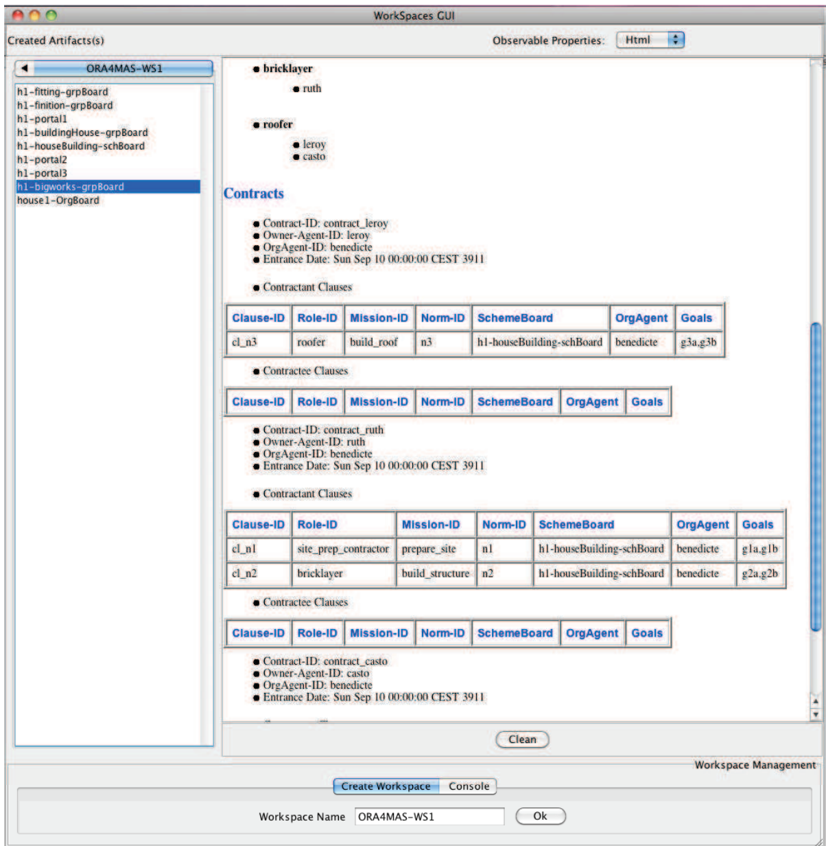
FIGURE E.11 – Gestion processus d'entrée : Contrats des agents Leroy et Ruth
