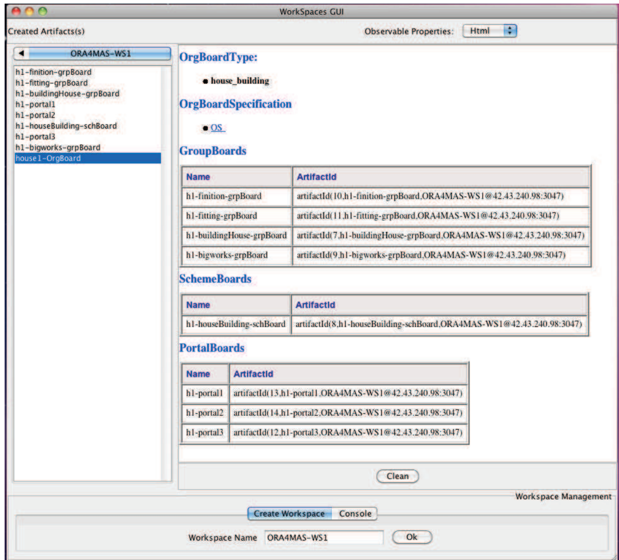
FIGURE E.1 – OrgBoard de l'entité organisationnelle : house1-OrgBoard
