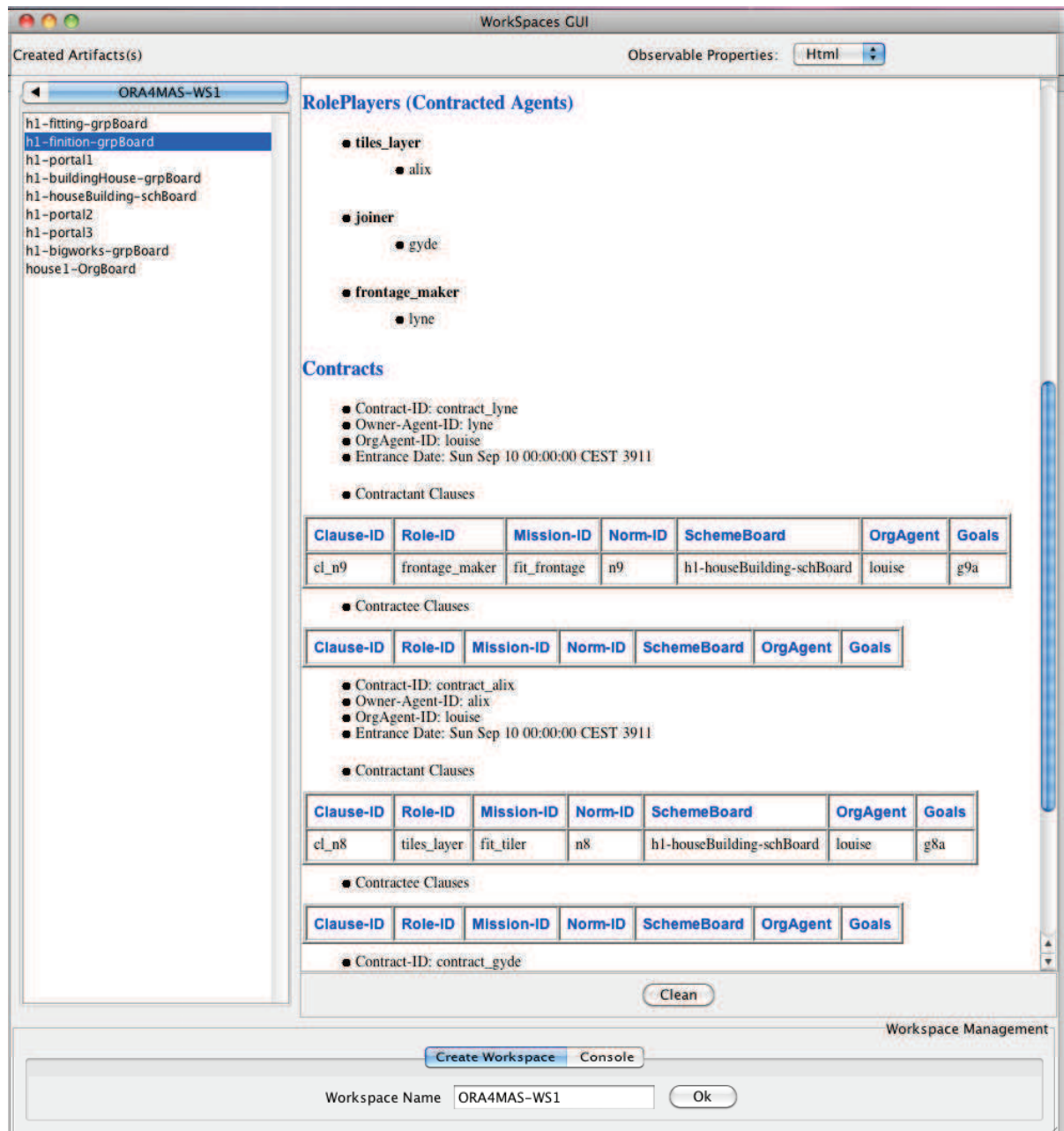
FIGURE E.12 – Gestion processus d'entrée : Contrats des agents Lyne et Alix
