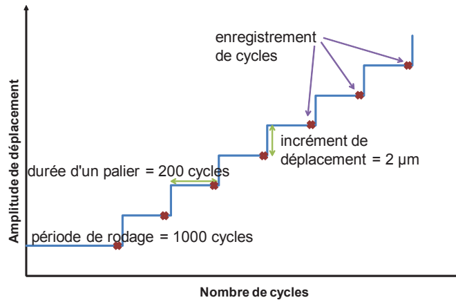
FIGURE 2.10 : Méthode des débattements variables
