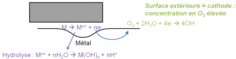
FIGURE 1.44 : Schéma des mécanismes de corrosion caverneuse dans les milieux chlorurés
