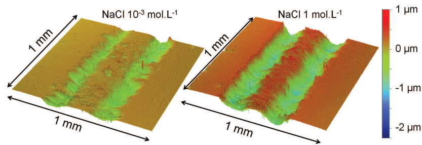
FIGURE 3.9 : Trace d'usure du 316L en forme de "W" après fretting, pour les solutions de NaCl 10^{-3} \text{ mol.L}^{-1} et 1 \text{ mol.L}^{-1} , zone de mesure = 1 \times 1 \text{ mm}
