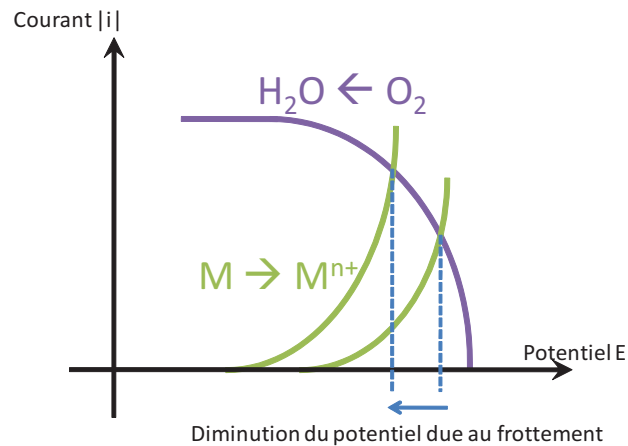
FIGURE 3.3 : Action du frottement : augmentation du courant anodique de dissolution \rightarrow diminution du potentiel mixte
