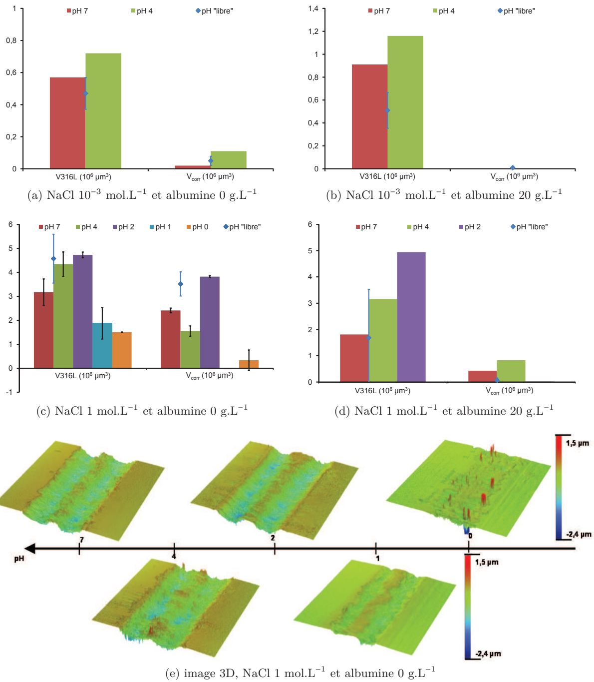
FIGURE 4.32 : (a), (b), (c), (d) Valeur du volume d'usure du 316L et du volume de corrosion à pH 7, pH 4, pH 2, pH 1 et pH 0, l'essai à pH "libre" est représenté par un \blacklozenge et (e) image 3D des traces d'usure en fonction du pH, image = 1 mm x 1 mm
