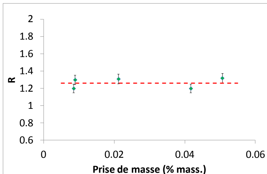
Figure 102. Résultats du test « \Phi.S_m » pour les décrochements en température de 780 °C à 800 °C à différentes prises de masse.
