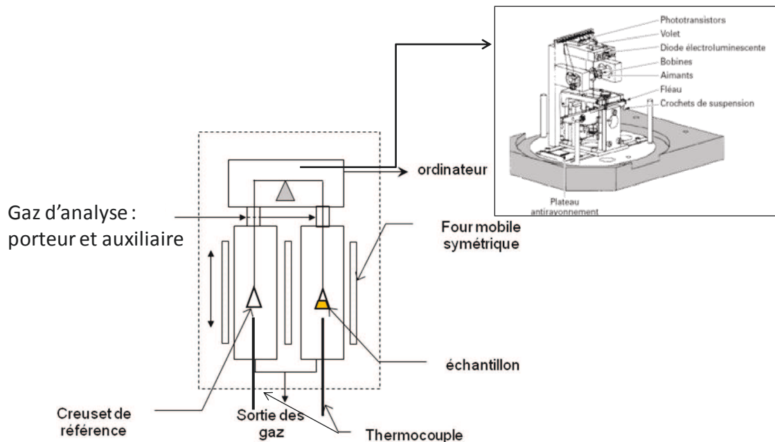
Figure 56: Schéma de la thermobalance TAG 16 de Setaram
