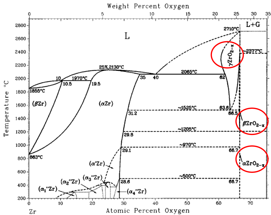
Figure 4. Diagramme de phase du système Zr-O [28].
