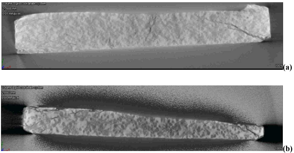
Figure 36. Coupes transverses du (a) cermet A, (b) cermet B frittés
