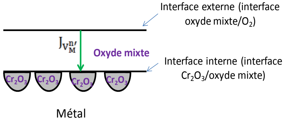
Figure 104. Schéma représentant l'oxydation externe du cermet
