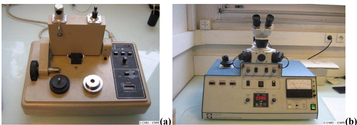
Figure 110. Préparation des pastilles destinées au MET : (a) dimpleur et (b) PIPS.
