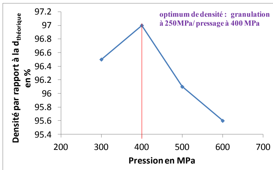
Figure 33. Courbe de densification (par poussée d'Archimède) du cermet A fritté à 1350 °C
