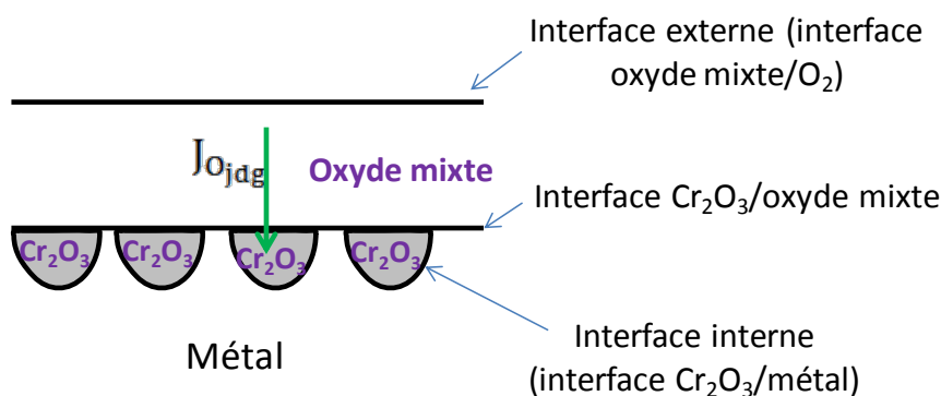
Figure 103. Schéma représentant l'oxydation interne du cermet
