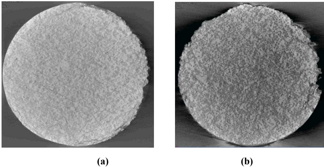
Figure 35. Coupes radiales du (a) cermet A et du (b) cermet B frittés
