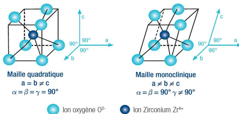
Figure 5. Schéma des structures cristallographiques quadratique et monoclinique de la zircone [24]
