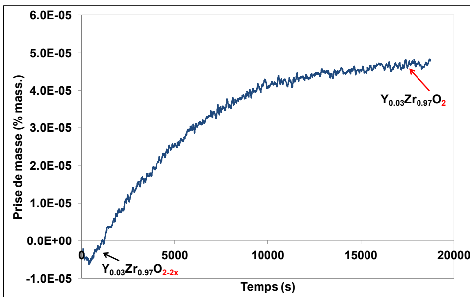
Figure 99. Analyse thermogravimétrique de la pastille frittée de ZrO_2 (TZ-3Y-E) oxydée à 800\text{ }^\circ\text{C} sous 20\text{ }\% O_2 pendant 6 heures
