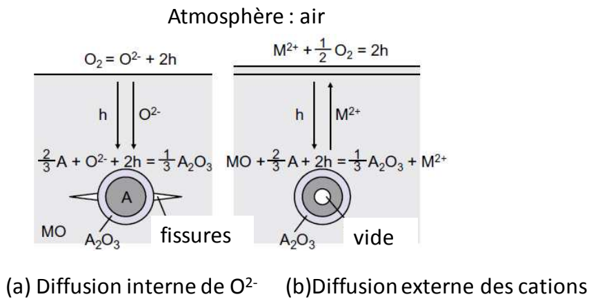
Figure 13. Schéma de la cinétique d'oxydation des M(p)-CMC(s) : (a) par diffusion anionique interne, (b) par diffusion cationique externe [46].
