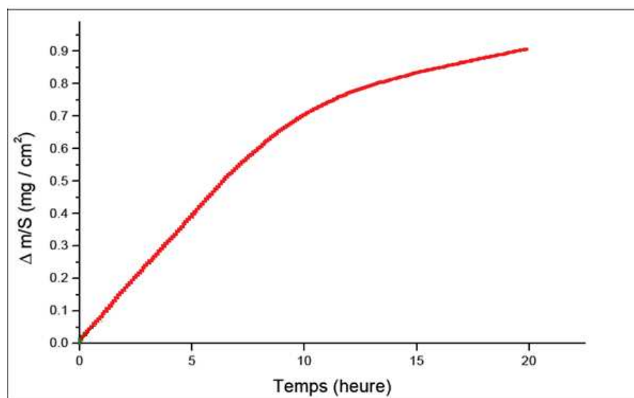
Figure 49. Prise de masse en fonction du temps d'une plaquette de 304L oxydé à 1000 °C sous air [92]
