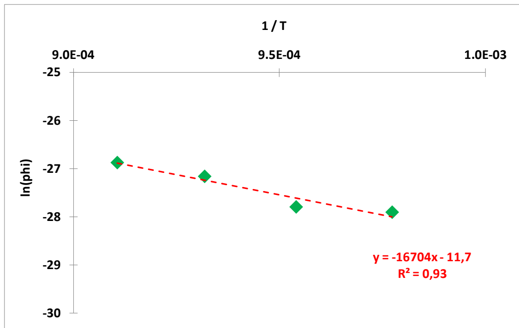
Figure 72. Variation de \ln \Phi en fonction de 1/T ( \text{K}^{-1} )
