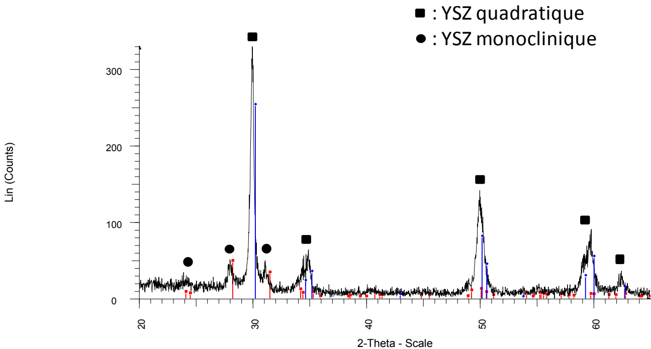
Figure 18. Diagramme de diffraction des rayons X (DRX) de la poudre TZ-3Y-E
