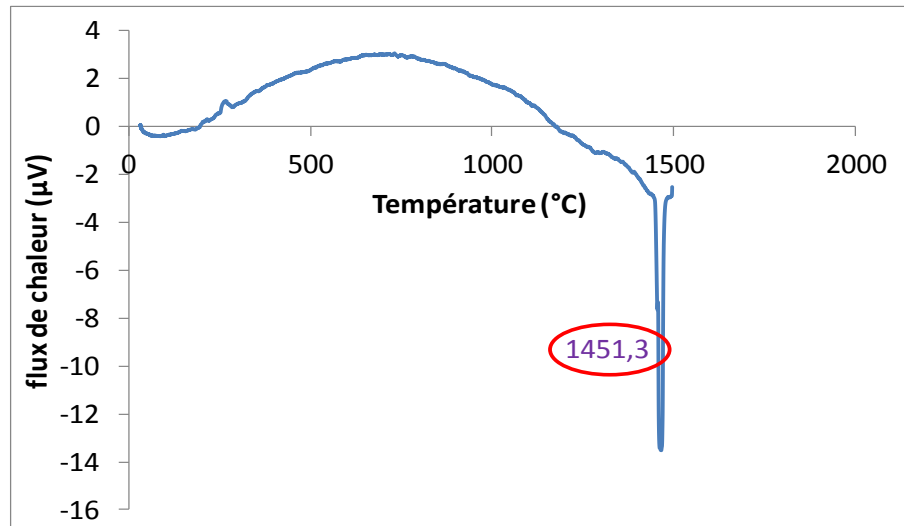
Figure 19. Analyse thermique différentielle de la poudre 304L
