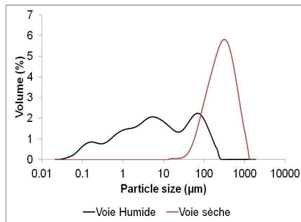
Figure 23. Granulométrie laser de la poudre du cermet
