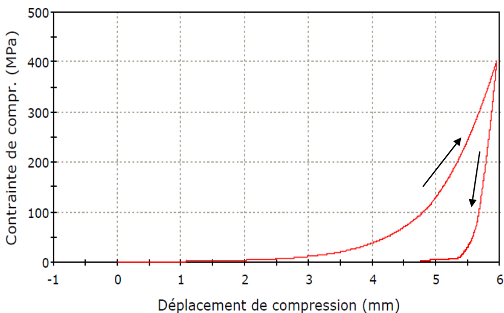
Figure 27. Courbe de compression de la poudre de cermet à 400 MPa
