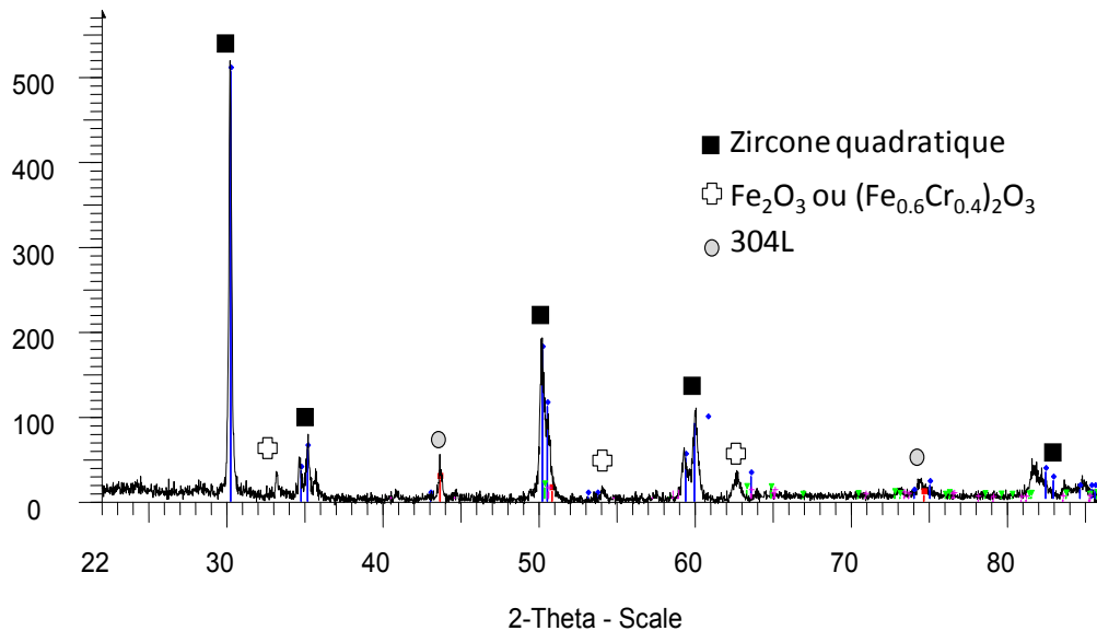
Figure 98. DRX du cermet A4 oxydé à 800 °C pendant 6 heures sous 20 % O 2
